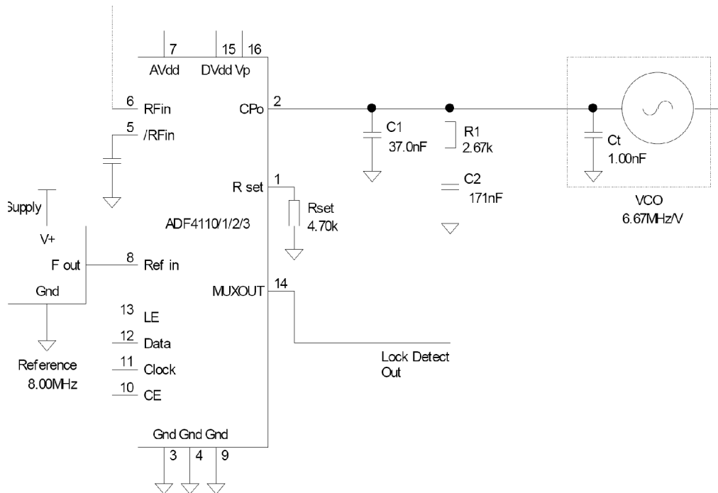
Obr. B.1: Schéma generované programem ADIsimPLL
