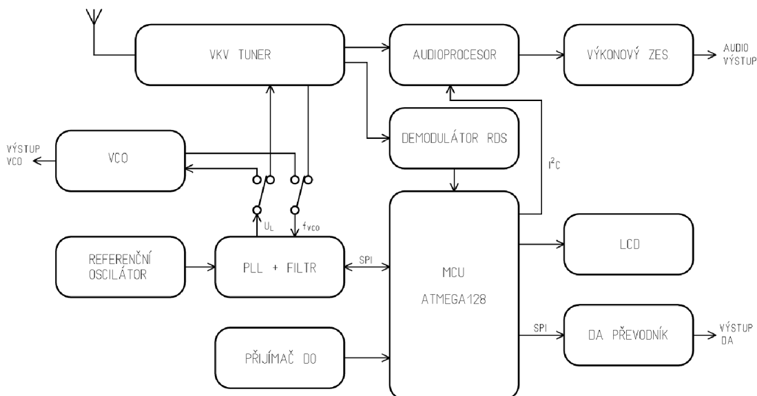
Obr. 2.1: Blokové schéma
