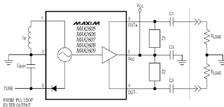
Obr. 2.4: Typické zapojení obvodu MAX2606 [10]
