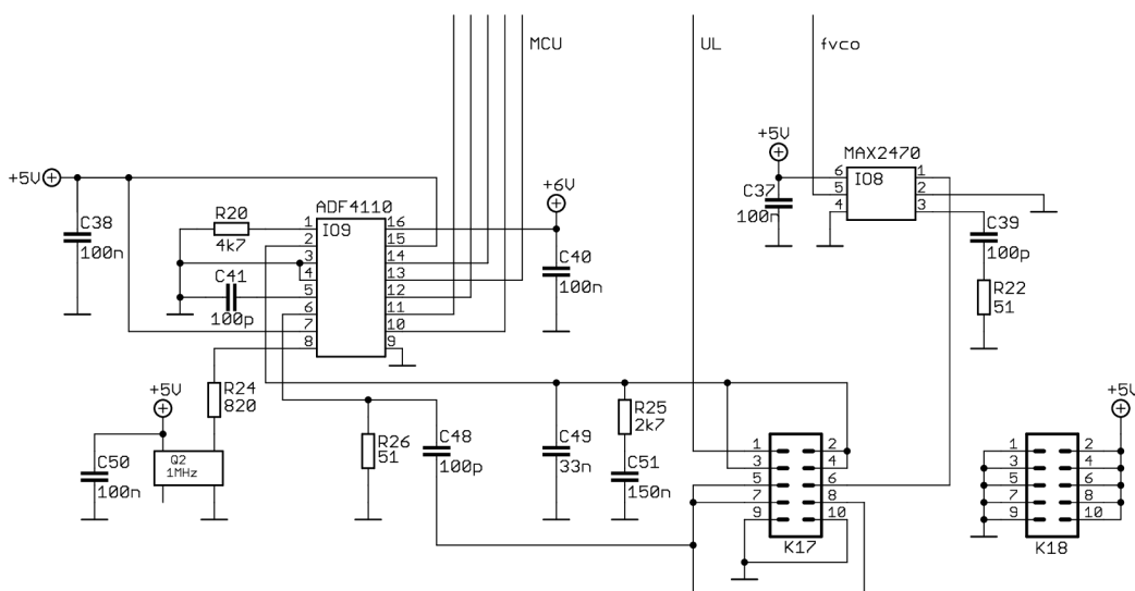
Obr. 3.1: Schéma obvodu fázového závěsu
