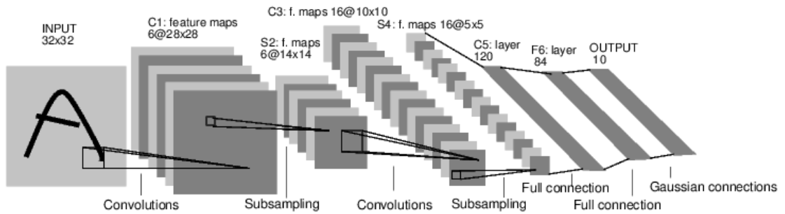
Obr. 4.2: Architektúra neurónovej siete LeNet-5. Neurónová sieť slúži na klasifikáciu písmen a čísel. Prevzaté z http://eblearn.sourceforge.net/beginner_tutorial2_train.html .
