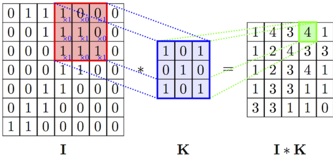
Obr. 5.1: Ilustrácia výpočtu konvolučnej vrstvy pri vstupe I a konvolučnom jadre K . Prezaté z https://cambridgespark.com/content/tutorials/convolutional-neural-networks-with-keras/index.html .
