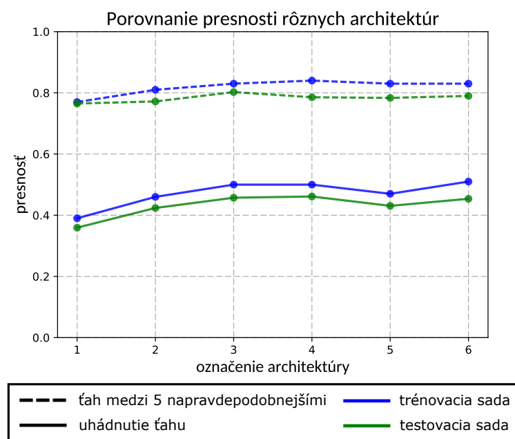
Obr. 7.5: Presnosť jednotlivých architektúr strategickej siete s tromi konvolučnými vrstvami na trénovacej a testovacej sade. Architektúry použitých neurónových sietí sú podrobne popísané v tabuľke 7.2.
