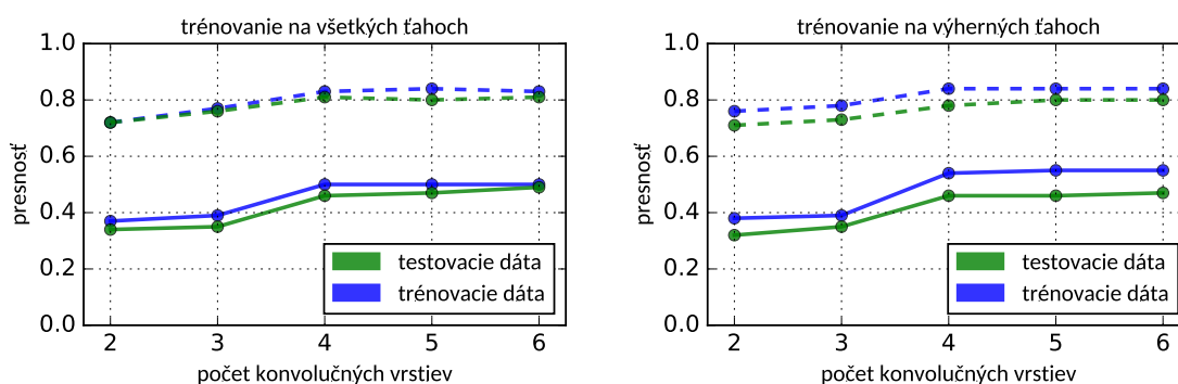
Obr. 7.4: Úspešnosť jednotlivých strategických sietí na testovacej a trénovacej dátovej sade. Plná čiara reprezentuje uhádnutie ťahu a prerušovaná, že hľadaný ťah bol medzi piatimi najpravdepodobnejšími. Kvôli nedostatočnej veľkosti trénovacej dátovej sady sú niektoré neurónové siete mierne pretrénované.
