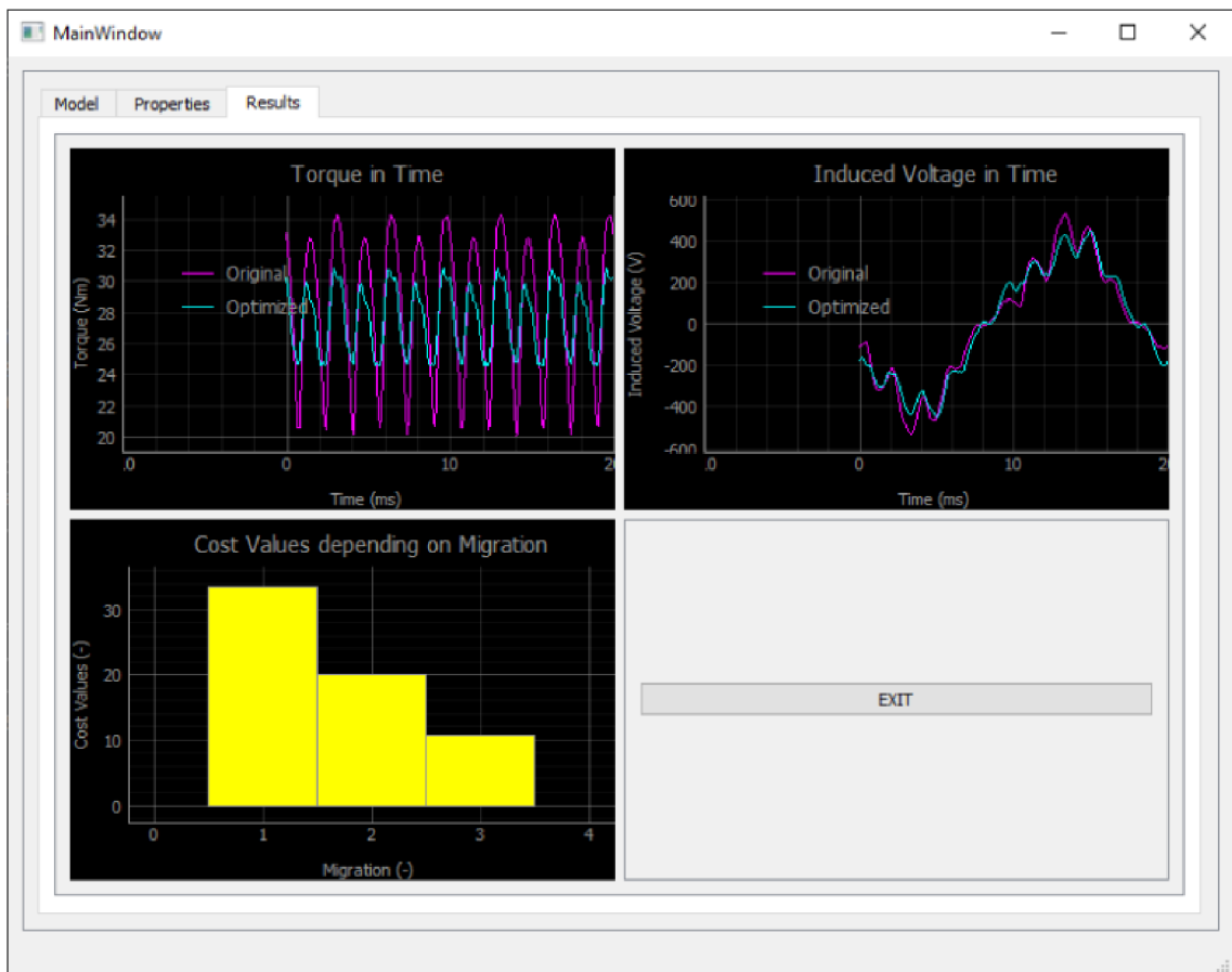
Obr. 6.2: Výsledek optimalizace
