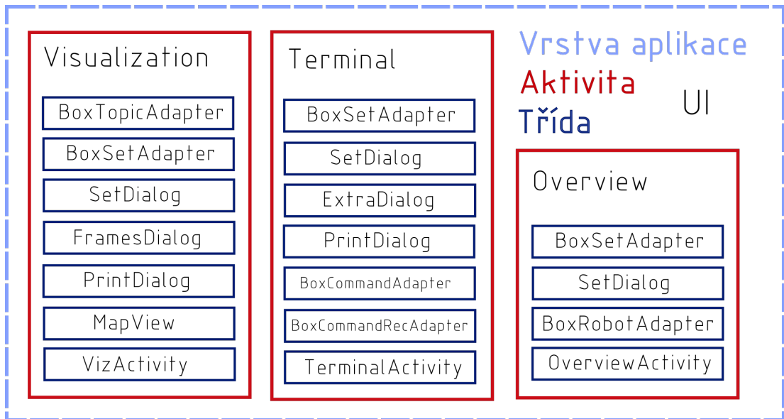
Obrázek 7.8: Třídy uživatelského rozhraní
