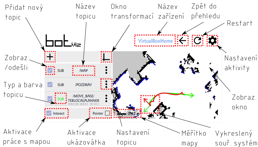
Obrázek 7.4: Vizualizace
