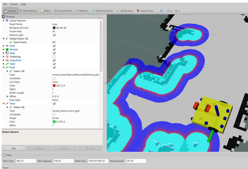
Obrázek 3.2: Prostředí RViz
