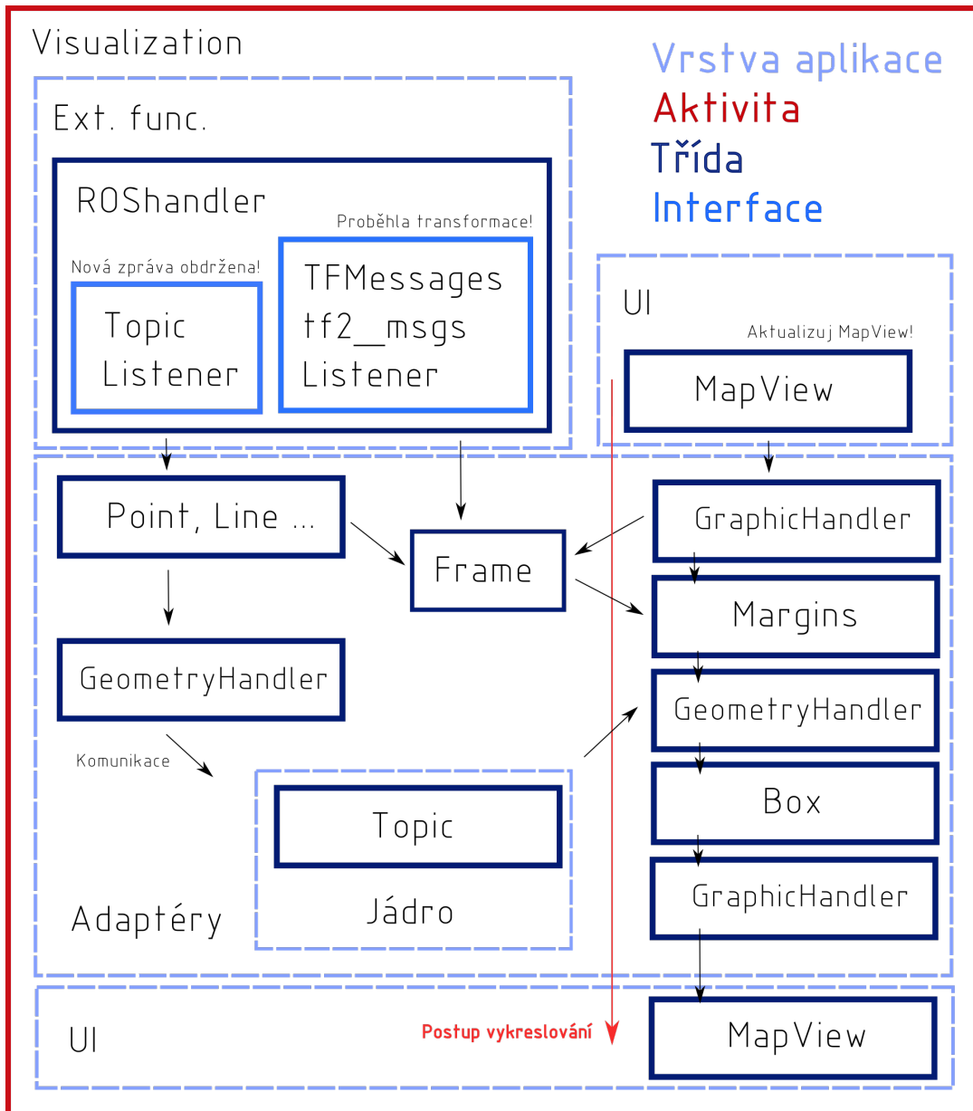
Obrázek 7.11: Vykreslování dat
