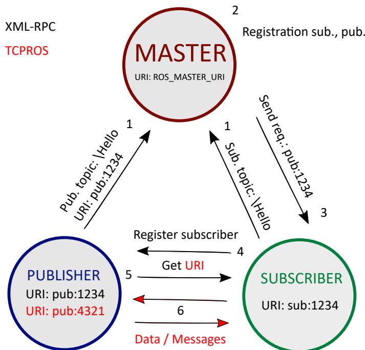
Obrázek 3.1: Schéma propojení Subscribera a Publishera [13, převzato, upraveno]
