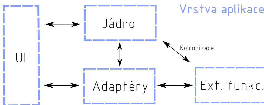
Obrázek 7.6: Struktura kódu
