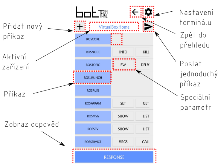
Obrázek 7.3: Terminálová aktivita
