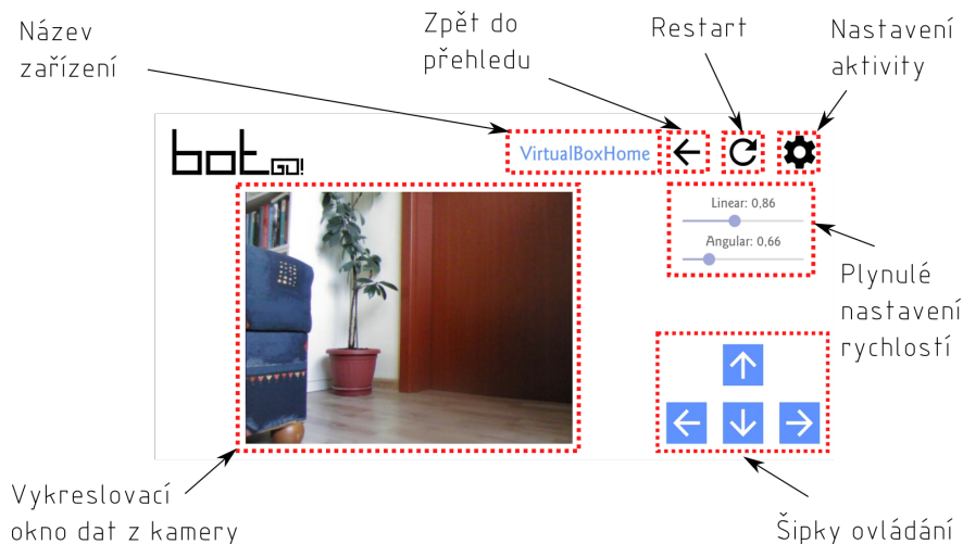
Obrázek 7.5: Aktivita Jed!
