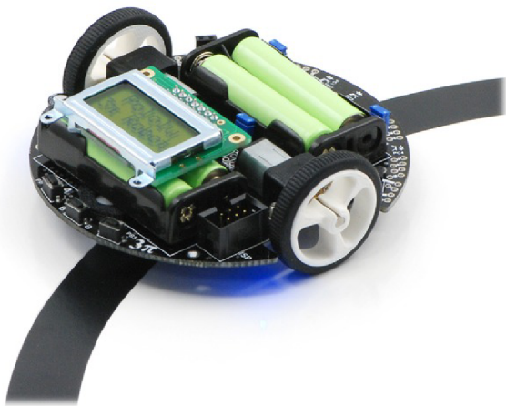
Obrázek 1.4: Robot Pololu 3pi 4
