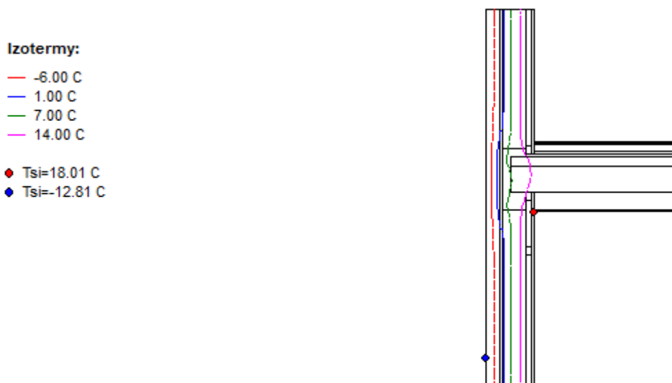
Obrázek 31: Grafický výsledek dvourozměrné simulace – Izotermy
