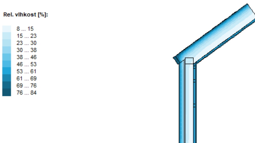
Obrázek 28: Grafický výsledek dvourozměrné simulace – relativní vlhkost
