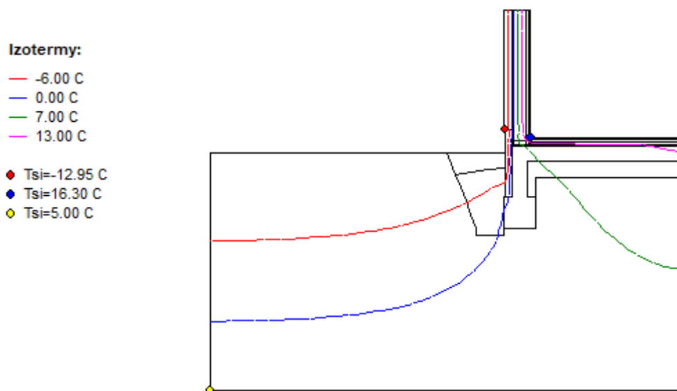
Obrázek 37: Grafický výsledek dvourozměrné simulace – Izotermy
