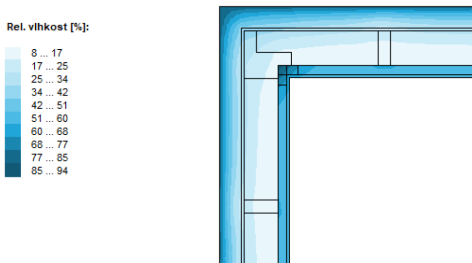
Obrázek 23: Grafický výsledek dvourozměrné simulace – relativní vlhkost
