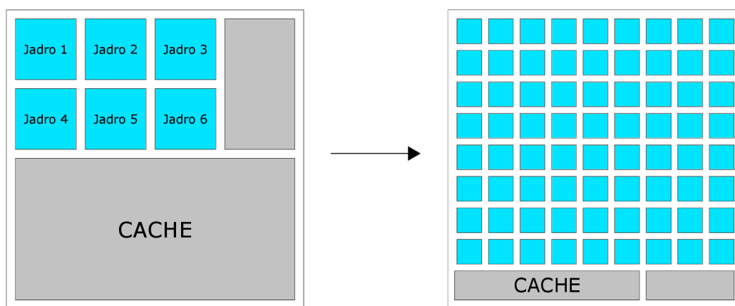
Obr. 3.2: Názorná ukážka rozdielneho využitia tranzistorov pri GPU. Značný počet tranzistorov sa uvoľnil vďaka možnosti zmenšiť cache. Ďalšie tranzistory sa uvoľnili vďaka nižšej náročnosti na výkon a mechanizmy jednotlivých jadier a teda vyžadujú menší počet tranzistorov. Tieto tranzistory je možné využiť pre pridanie nových jadier za účelom zvýšenia potencionálnej priepustnosti.
