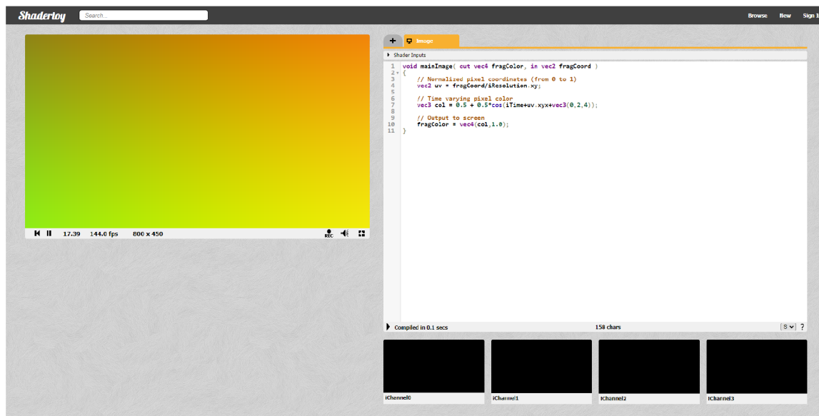
Obr. 2.1: Užívateľské rozhranie nástroja Shadertoy. V ľavej časti je možné vidieť náhľad spustenej aplikácie. V pravej časti sa nachádza editor kódu a tlačidlá pre špecifikáciu vstupov.
