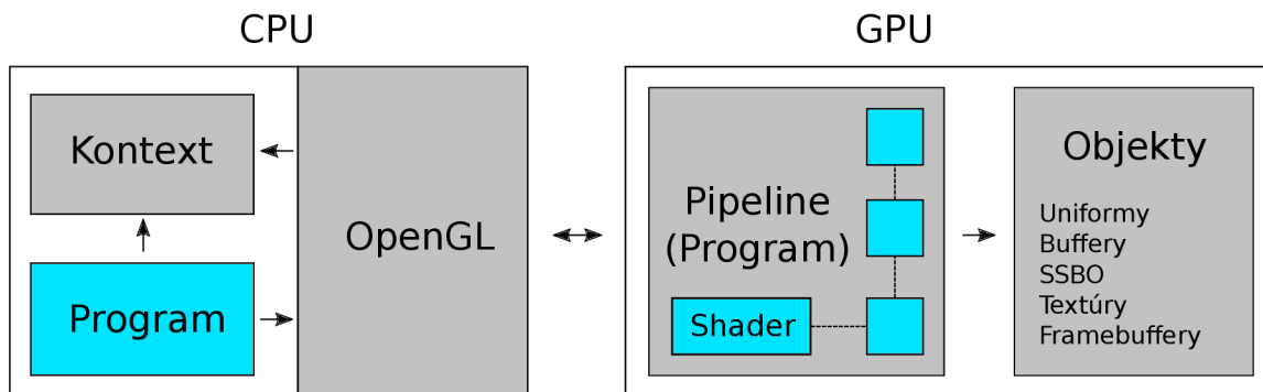
Obr. 3.5: Znázornenie akým spôsobom funguje OpenGL. Program bežiaci na CPU využíva OpenGL API pre komunikáciu s GPU. Aktuálny stav je uložený v kontexte OpenGL. Interné procesy GPU (pipeline) je možné programovať pomocou shaderov. Jednotlivé shadery počas behu prístupujú k objektom, ktorých dáta sú typicky uložené vo VRAM a ich stav v kontexte.
