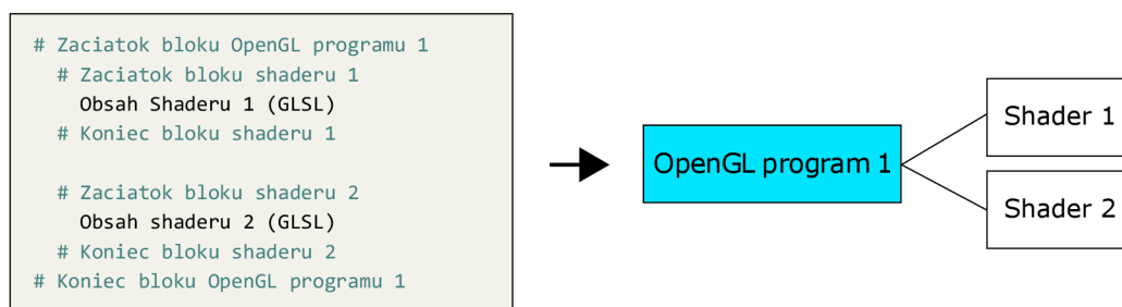
Obr. 4.1: Znázornenie štruktúry zdrojového kódu aplikácie. Pomocou deklarácií začiatku a konca bloku môže engine spätne skonštruovať jednotlivé OpenGL programy a priradiť im ich shadery. V rámci deklarácie začiatku bloku shaderu musí byť špecifikovaný aj jeho typ.
