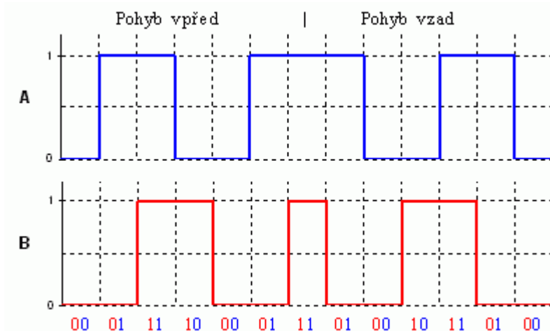
Obrázek 10 Inkrementální enkodér
