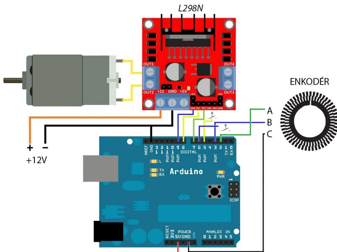
Obrázek 18 Zapojení obvodu
