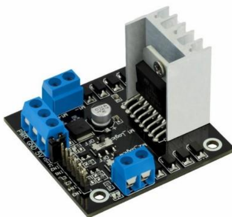
Obrázek 8 H-můstek L298N
