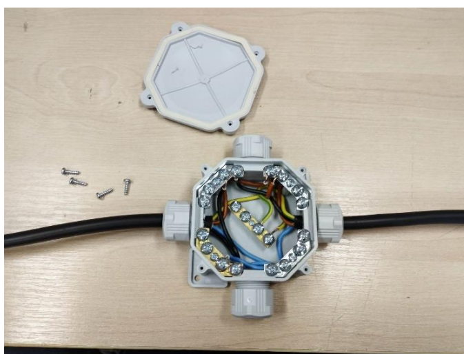
Obrázek 7: Otevřená krabice ACIDUR s praktickým propojením svou kabelů CYKY 4Cx 1,5 mm Zdroj: Vlastní fotografie
