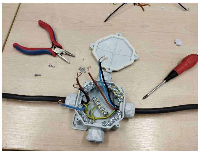
Obrázek 6: Otevřená krabice ACIDUR s napodobením výroby oček Zdroj: Vlastní fotografie
