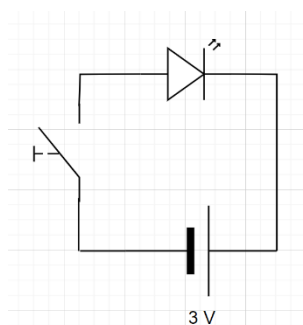
Obrázek 10: Schéma zapojení obvodu k hůlce z HP
