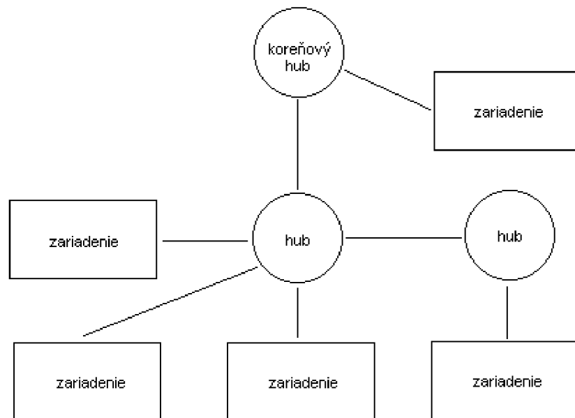
Obrázek 1: Topológia USB
