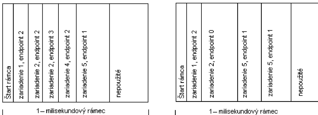
Obrázek 2: Schéma prenosových rámcov
