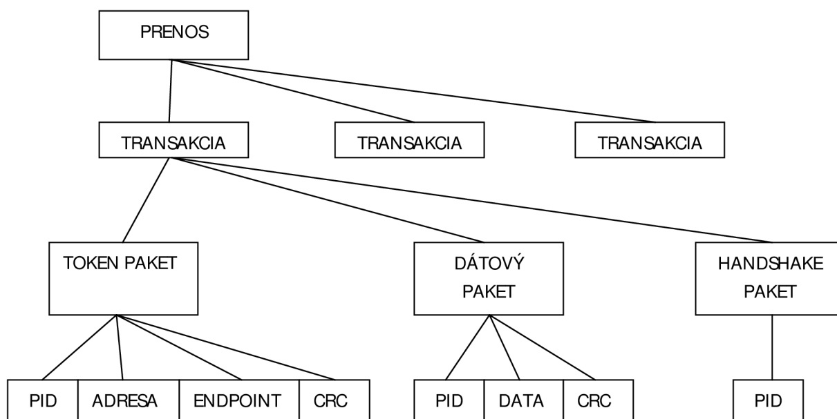
Obrázek 4: Hierarchia prvkov prenosu
