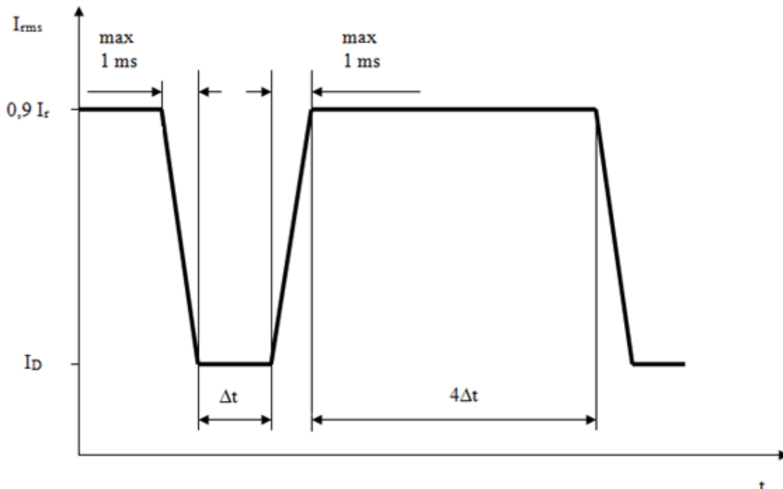
Obrázek 9.1: Zkušební proud [11]
