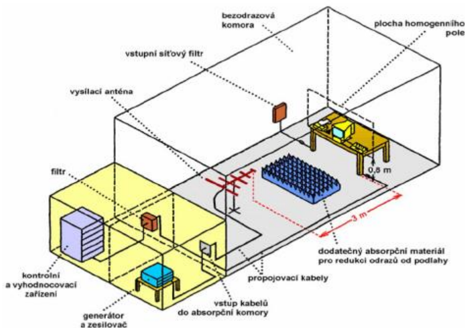
Obrázek 4.4: Zkušební laboratoř pro zkoušku vyzařovaným vysokofrekvenčním elektromagnetickým polem [1]
