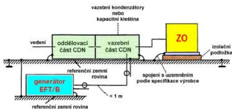
Obrázek 5.3: Uspořádání pracoviště [1]
