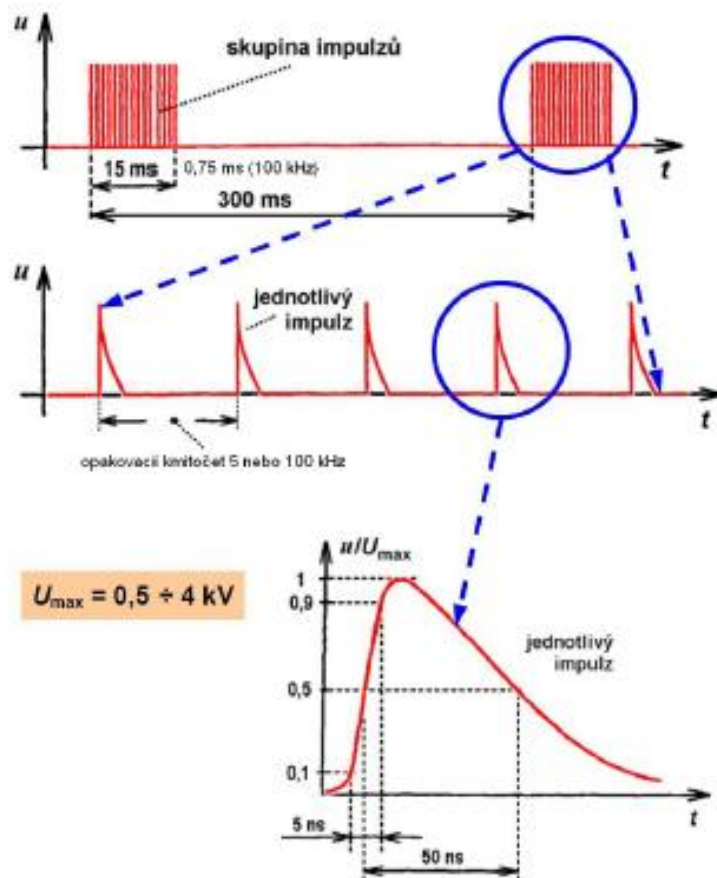
Obrázek 5.1: Zkušební signál [1]
