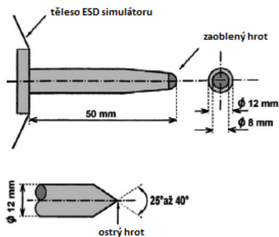
Obrázek 10.5: Zkušební hroty
