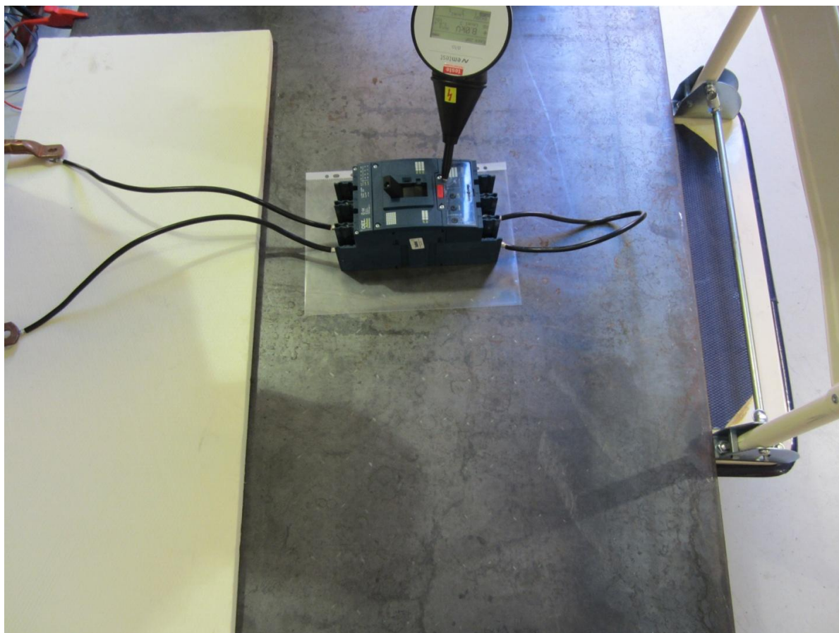
Obrázek 10.6: Zkouška přímým kontaktním elektrostatickým výbojem
