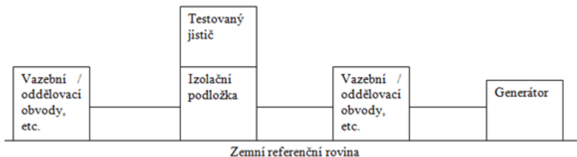
Obrázek 7.1: Znázornění rozmístění zařízení během zkoušky [16]
