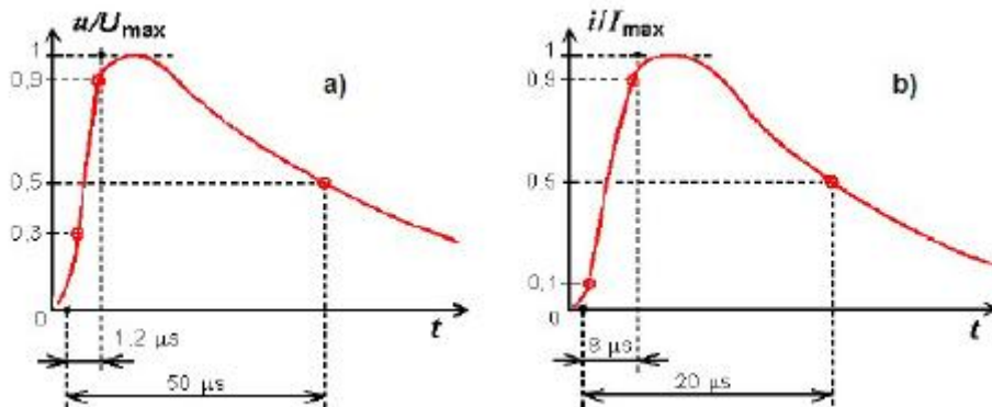
Obrázek 6.1: Zkušební rázová vlna: a) napět'ová naprázdno, b) proudová nakrátko [1]
