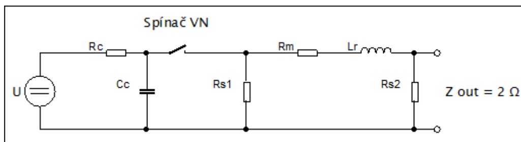
Obrázek 6.2: Principiální schéma zapojení generátoru kombinované vlny [1, 15]
