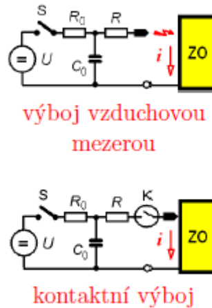
Obrázek 10.4: Zjednodušené zapojení zkoušek odolnosti vůči ESD; ZO – zkoušený objekt [1]
