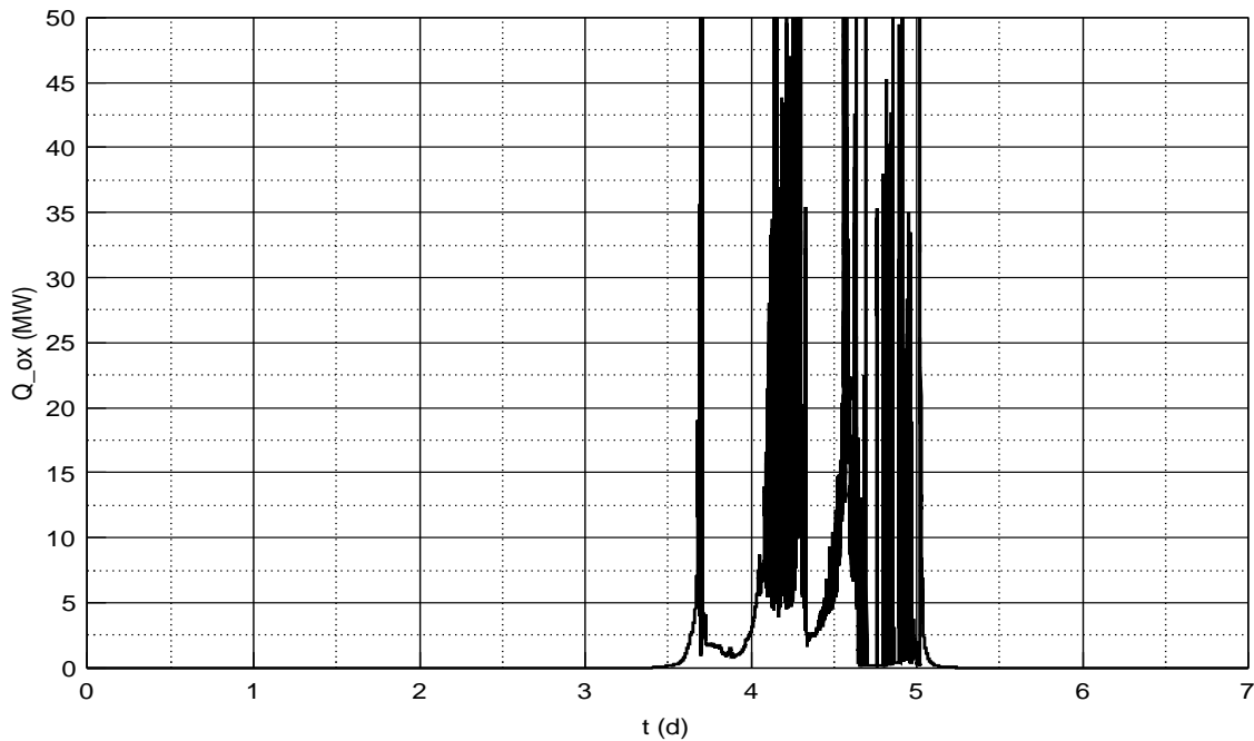
Obr. 5.4: Okamžitá hodnota generovaného oxidačného tepla pri poruche so stratou chladienia
