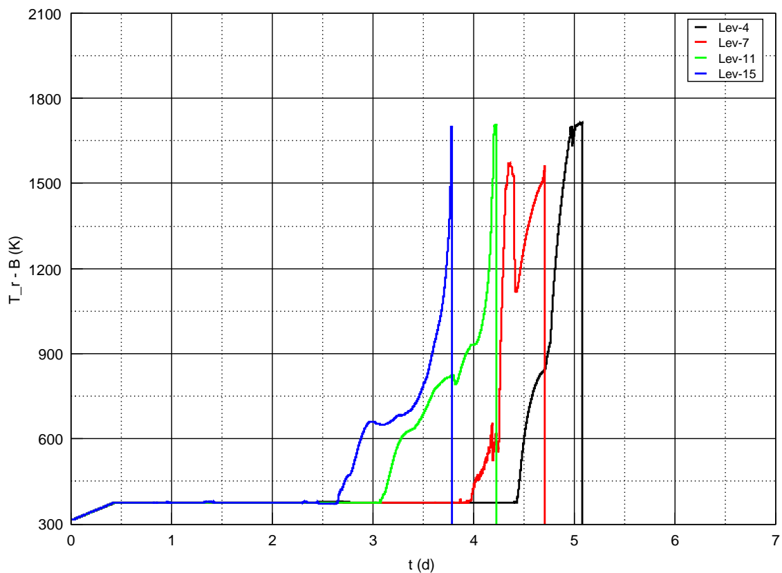
Obr. 5.3: Teplota roštov pri poruche so stratou chladienia
