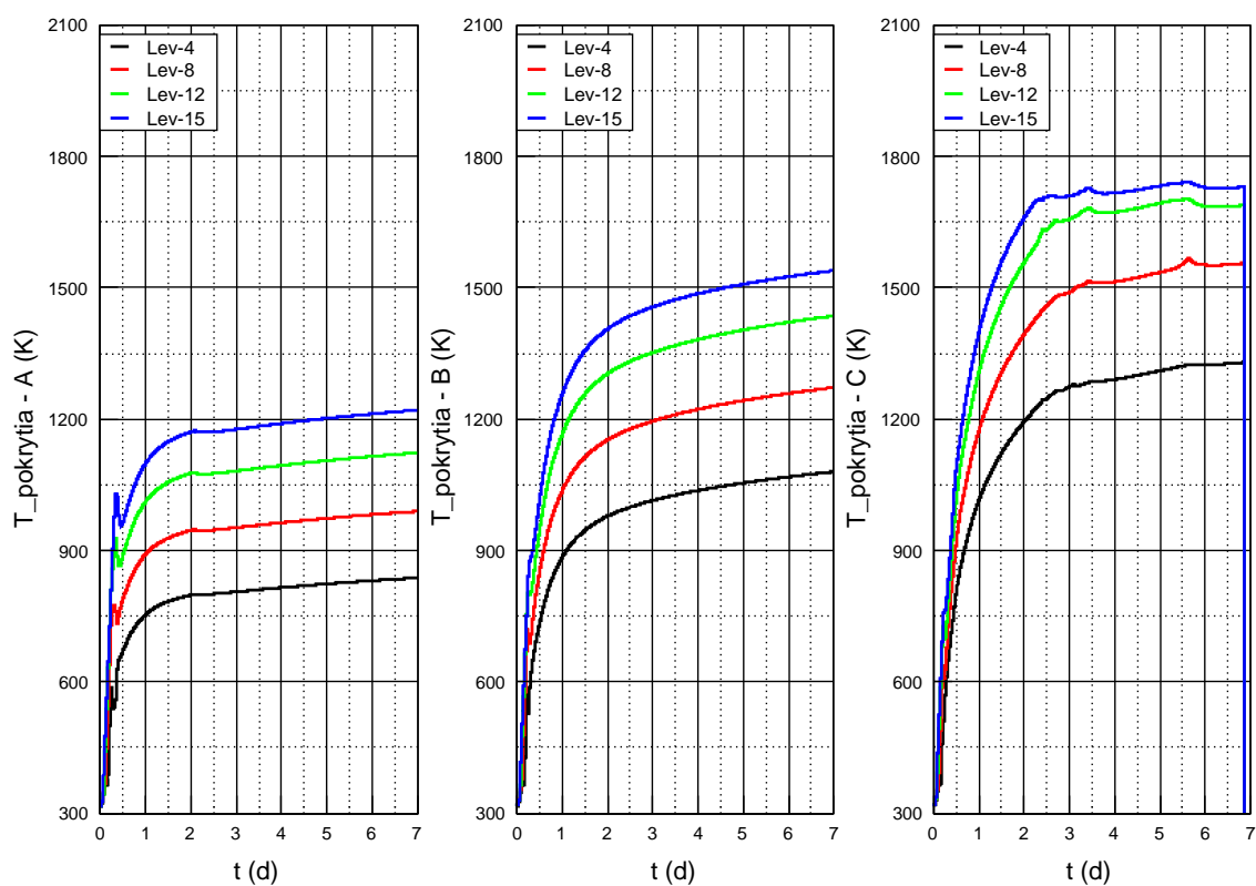
Obr. 5.11: Teplota pokrytia pri poruche so stratou chladiva: A)zvýšená ventilácia, B)pôvodná ventilácia C)žiadna ventilácia
