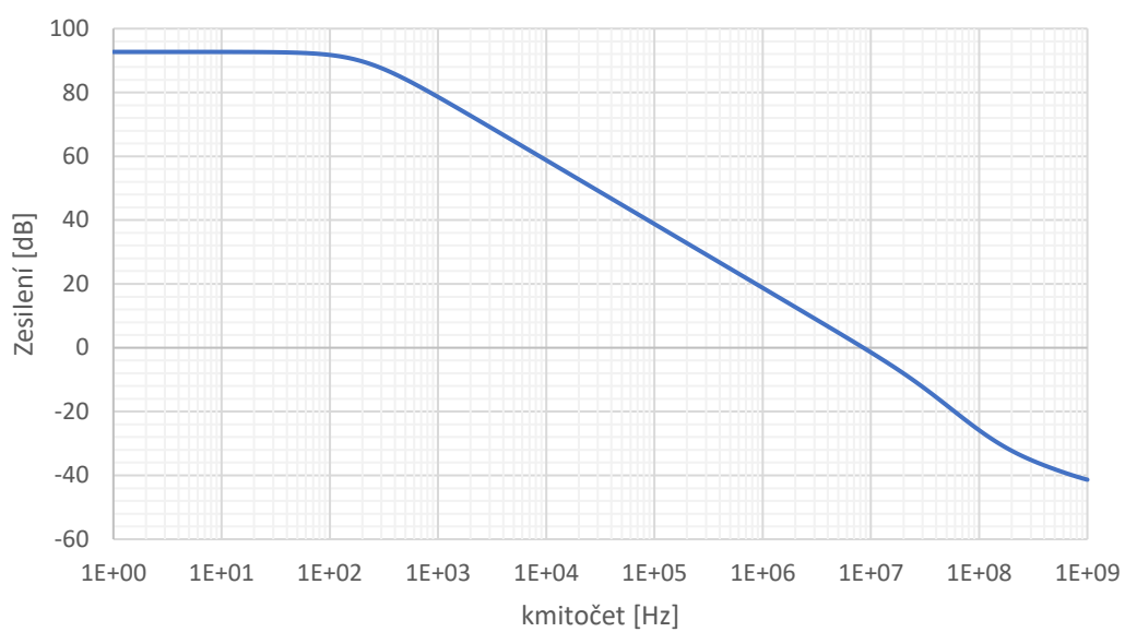
Obrázek 3.11: Amplitudová kmitočtová charakteristika dvoustupňového OZ
