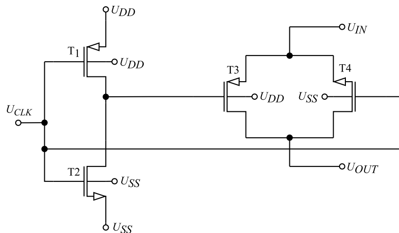
Obrázek 2.6: Základní spínač MOS využívající komplementárního zapojení
