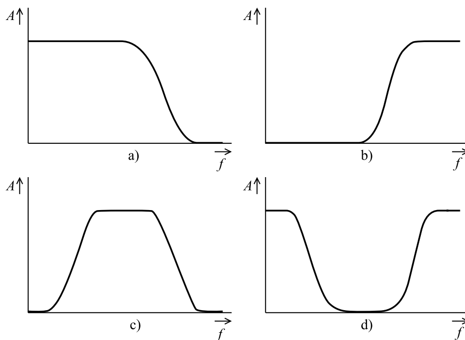
Obrázek 1.2: Průběh závislosti zisku na kmitočtu, a) dolní propust, b) horní propust, c) pásmová propust, d) pásmová zadrž
