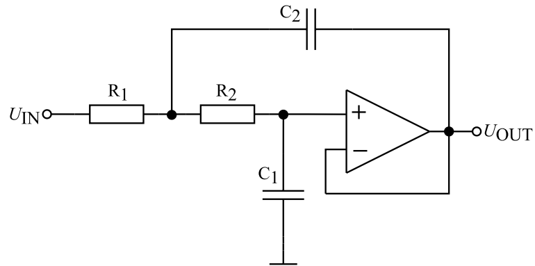
Obrázek 4.1: Sallen–Key filtr
