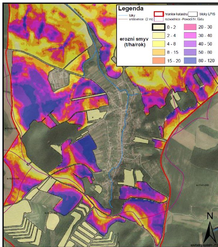
Obr. 3. 4. 6 Rastrové zobrazení průměrné roční sumy erozního smyvu pro R faktor 50
