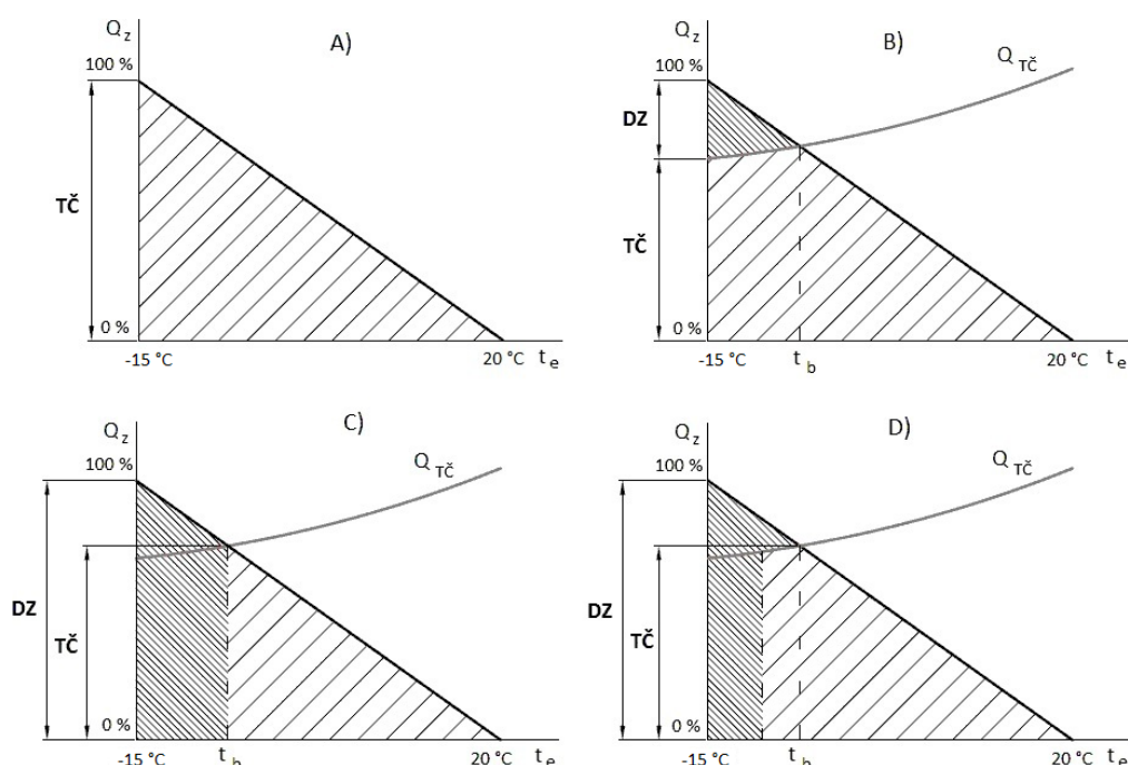
Obrázek 1.2 Grafy závislosti tepelných ztrát na venkovní teplotě: [6]
