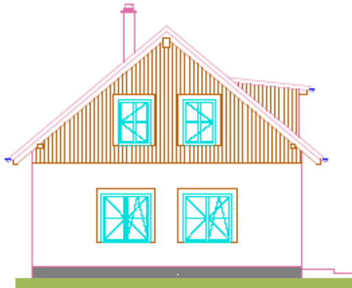
SEVEROZÁPADNÍ POHLED
