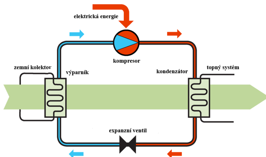
Obrázek 1.1 Princip práce tepelného čerpadla, převzato z [3], upraveno autorem
