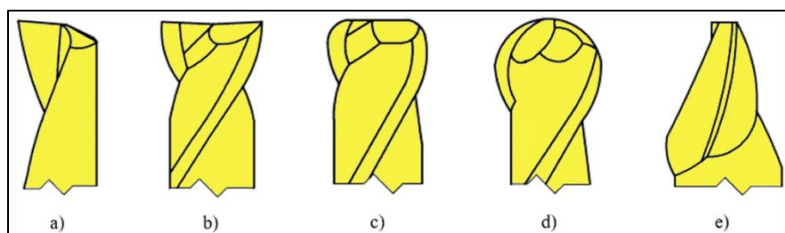
Obr. 2.12 - Schematické znázornění stopkových mikrofréz: a) jednobřitá čelní, b) dvoubřitá čelní, c) čelní s rohovým rádiusem (toroidní), d) kulová, e) kuželová mikrofréza [6]
