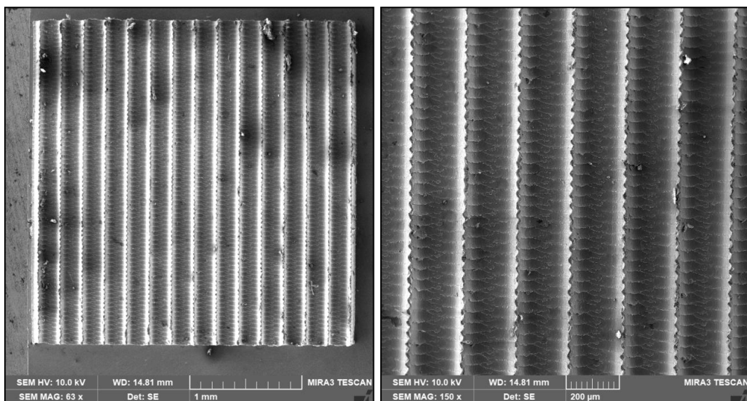
Obr. 4.16 - SEM snímky obrobeného reliéfu vzorku č. 2
