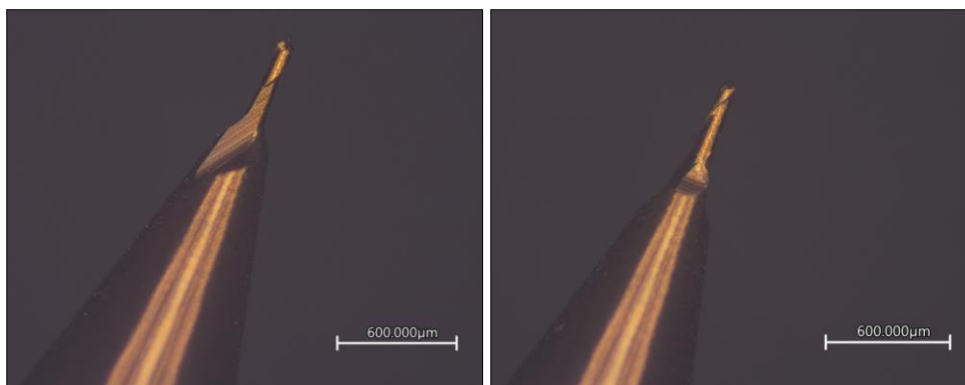
Obr. 3.2 - Detail řezné části nového nástroje, vyfoceno mikroskopem KEYENCE VK-X1000, zvětšení: 5x
