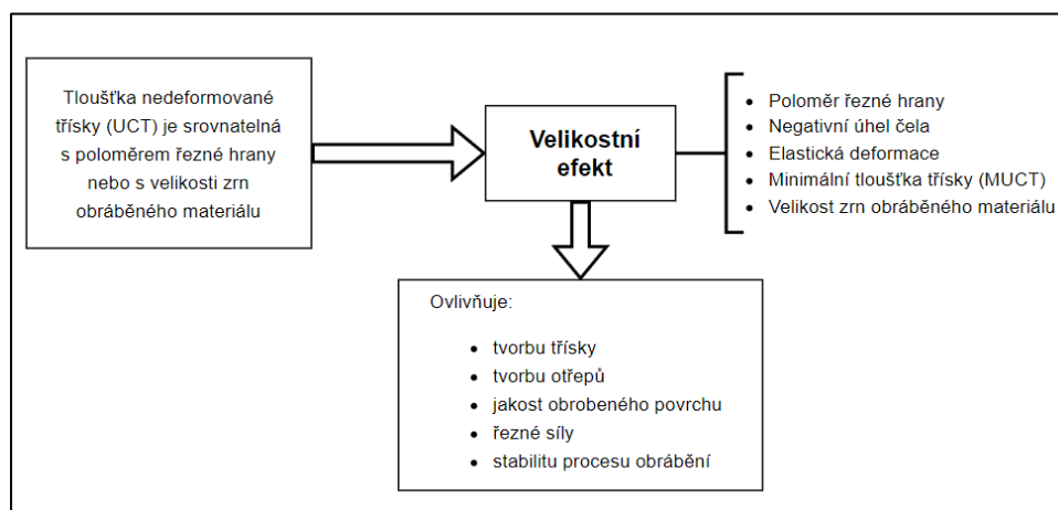
Obr. 2.8 – Velikostní efekt – co ho způsobuje a co ovlivňuje [3]
