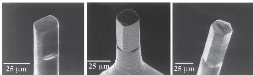
Obr. 2.11 - Mikrofrézy, o průměru 25 \mu\text{m} a poloměrem břitu menší než 0,1 \mu\text{m} , se (zleva) dvěma, čtyřmi a šesti řeznými hrany; vyrobené pomocí metody fokusovaného laserového paprsku [1]
