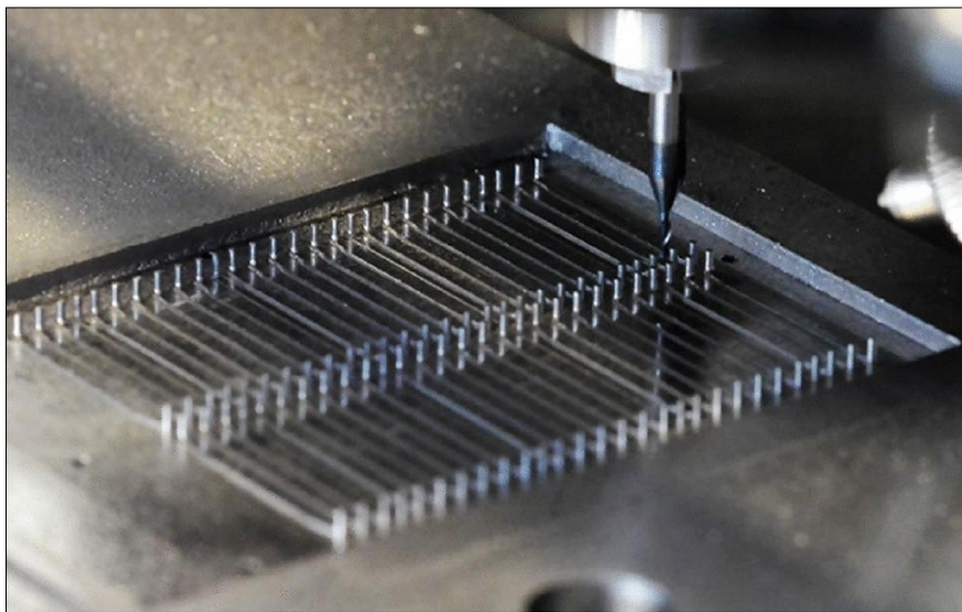
Obr. 2.1 - Mikrofluidní forma: 4 pole po 28 kolících o průměru 0,8 mm a výšce 2 mm [2]
