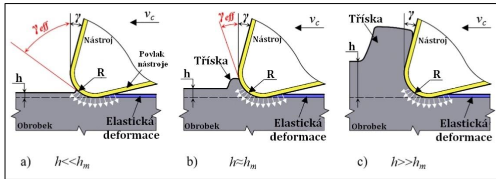
Obr. 2.7 – Schéma mechanismů úběru mikrotríscky: a) nedeformovaná tloušťka třísky ( h ) je menší než minimální nedeformovaná tloušťka třísky ( h_m ), b) hodnota h je srovnatelná jako hodnota h_m , c) hodnota h je větší než h_m [6]
