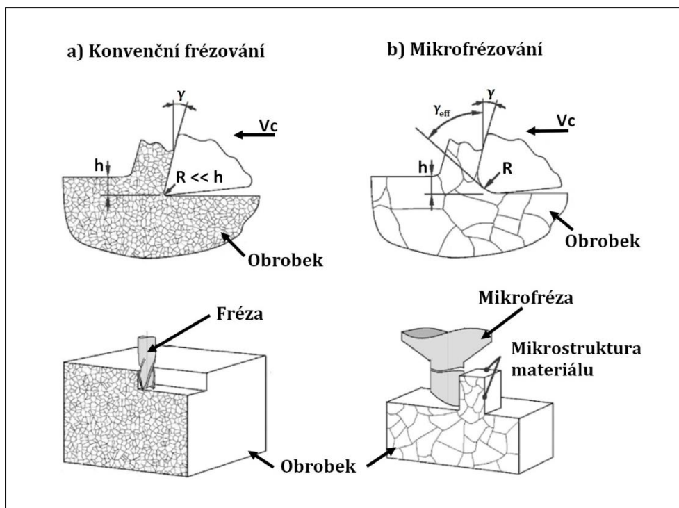
Obr. 2.5 – Znázornění a porovnání velikosti struktury obráběného materiálu u konvenčního frézování a mikrofrézování, vyplývající velikostní efekt způsobený vlivem zmenšení poloměru řezného nástroje, který je srovnatelný s tloušťkou nedeformované třísky či velikostí zrn obráběného materiálu [3]
