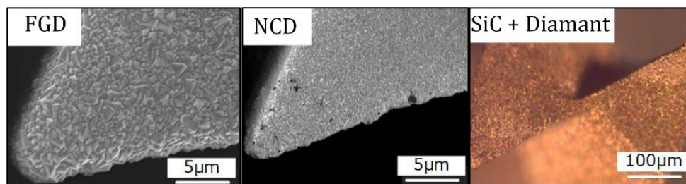
Obr. 2.19 – Diamantové povlaky: FGD (jemnozrný diamant), NCD (nanokrystalický diamant) a dvouvrstvý povlak SiC s diamantem. [3]
