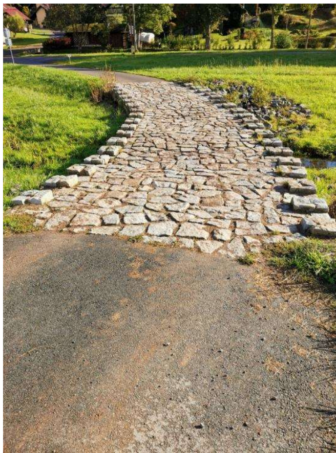
Obrázek 5: PBPO Vyvýšený brod pro přejezd aut a zemědělské techniky v obci k.ú. Písečná (zdroj autorka 2022).
