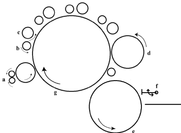
Obrázek 3 – Schéma válcového mykacího stroje; a – podávací válce, b – obraceč, c – pracovní válec, d – volant, e – snímací válec, f – sčesávací pilka, g – tambur
