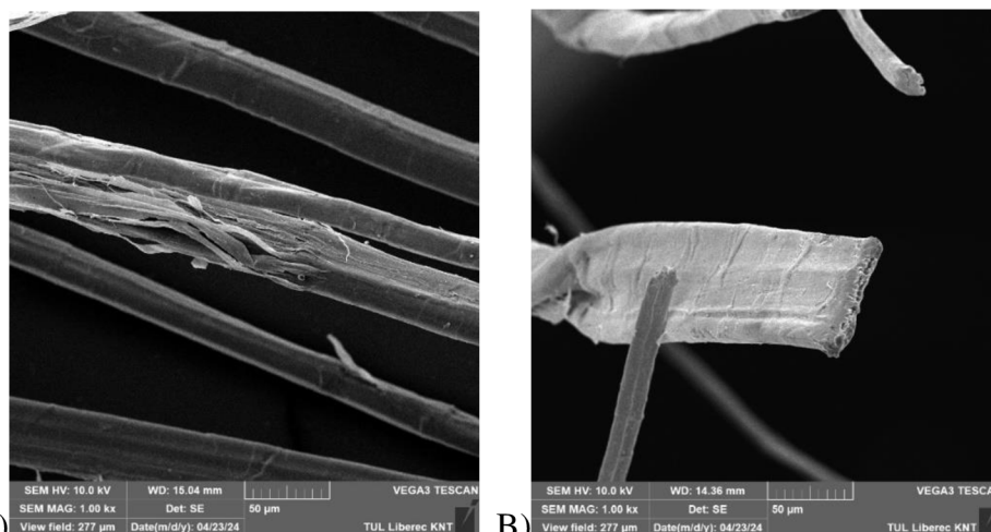
Obrázek 7 – Snímky banánových vláken z SEM zvětšení 1000×; A – Podélný pohled na vlákna a elementární vlákna, B – Sřih vlákn
