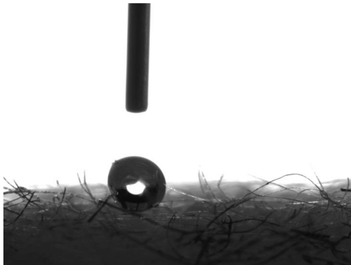
Obrázek 9 – Měření kontaktního úhlu banánových textilií
