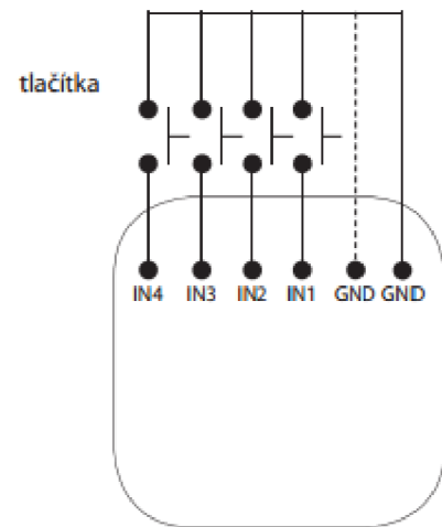
Obr. 4-10 Typové zapojení převodníku kontaktu RFIM-20B/40B/40B [10]
