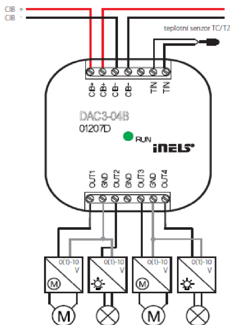
Obr. 4-14 Příklad zapojení A/D převodníku DAC3-04B [10]
