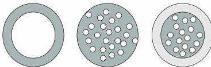
Obrázek 7: Možnosti enkapsulace [38]
