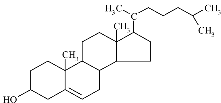
Obrázek 12: Cholesterol [51]
