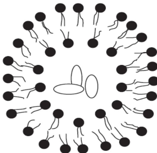
Obrázek 11: Liposom [32]
