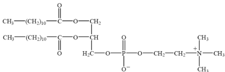
Obrázek 13: Lecithin [53]
