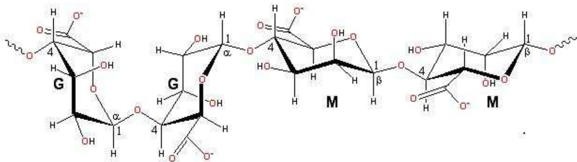
Obrázek 10: Struktura alginátu [47]
