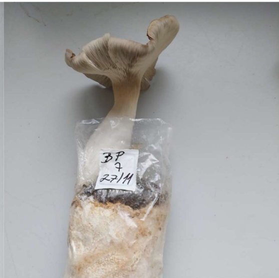
Obrázek č. 14: Plodnice na povrchu substratu kryté zeminou
