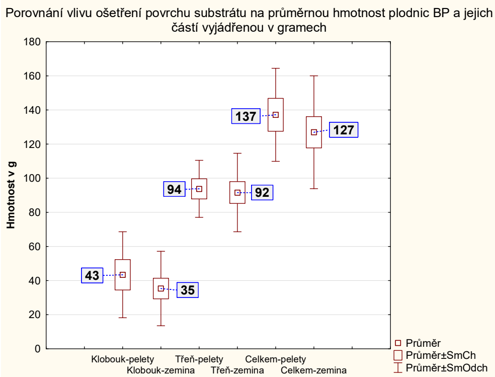
Graf č.5.2: Porovnání vlivu ošetření povrchu substrátu na průměrnou hmotnost plodnic BP a jejich částí vyjádřenou v g
