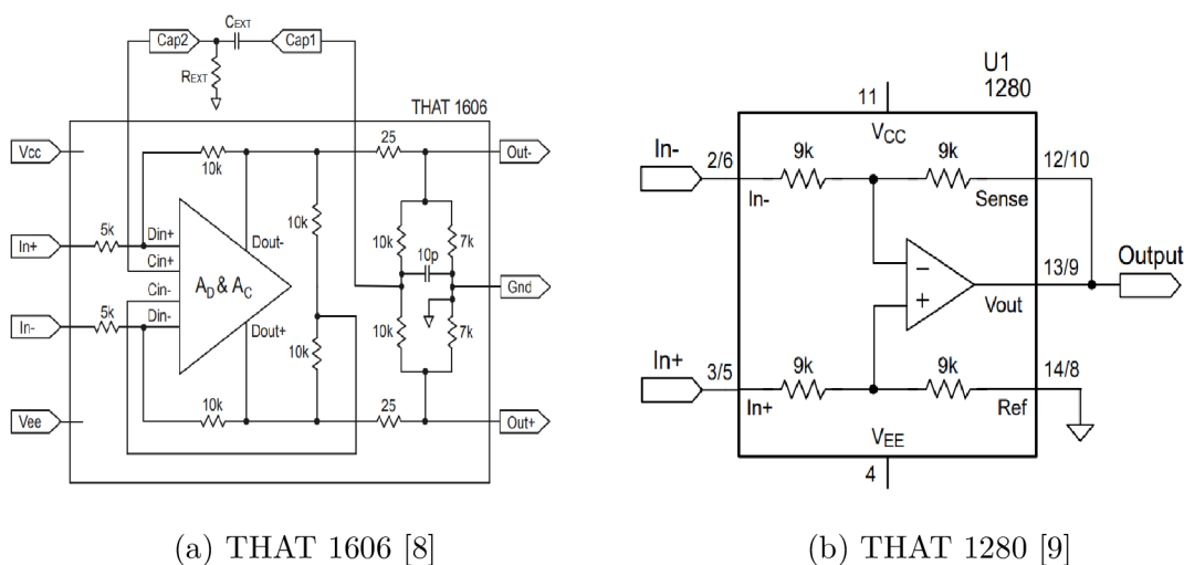
Obr. 1.4: Blokové schéma linkových obvodů
