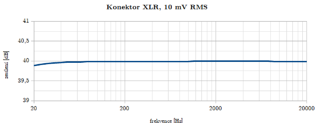
Kmitočtová charakteristika symetrického mikrofonního předzesilovače
