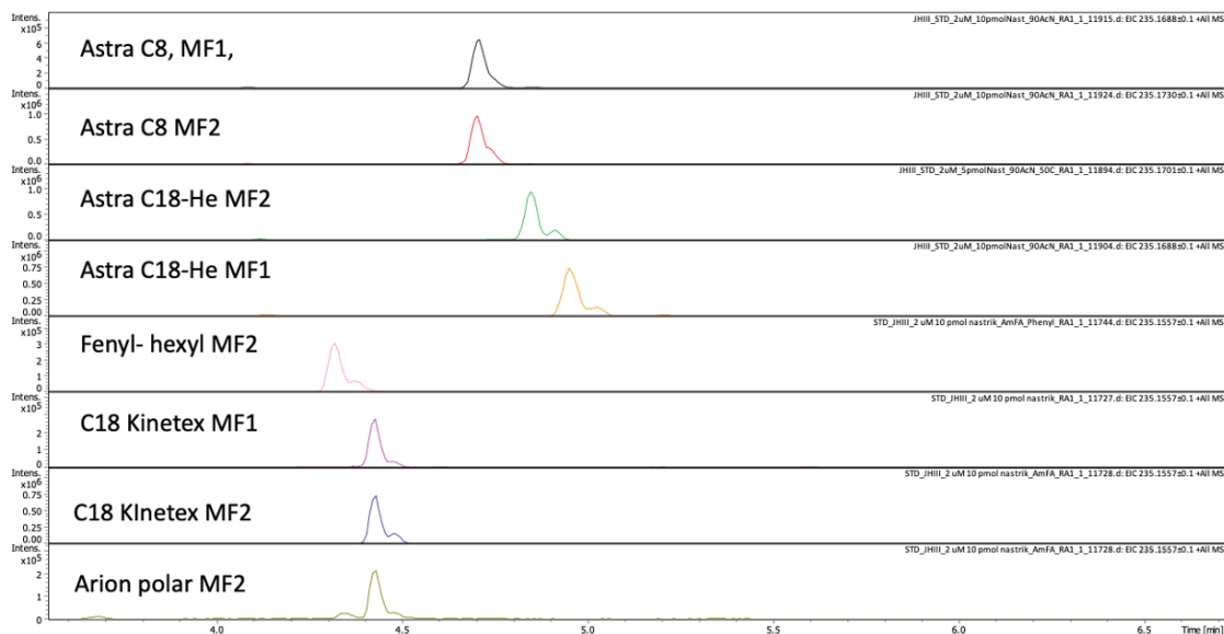
Obrázek 10 Extrahované chromatogramy pro fragment m/z 235,17 pro jednotlivé kolony za použití MF1 (FA) nebo MF2 (AmFA + FA). Nástřik JH III byl 10 pmol.
