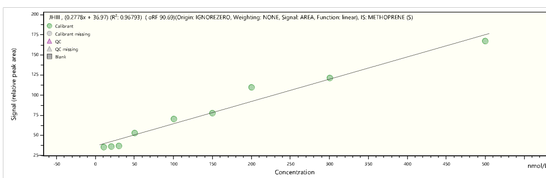
Obrázek 21 Kalibrační křivka č. 2 (Dry) Kalibrační řada byla připravena napipetováním JH III a MP o příslušných koncentracích do skleněných vialek. Směs se nechala odpařit v rotační vakuové odparce a vzniklý odparek se resuspendoval v 50 \mu l 90% acetonitrilu.
