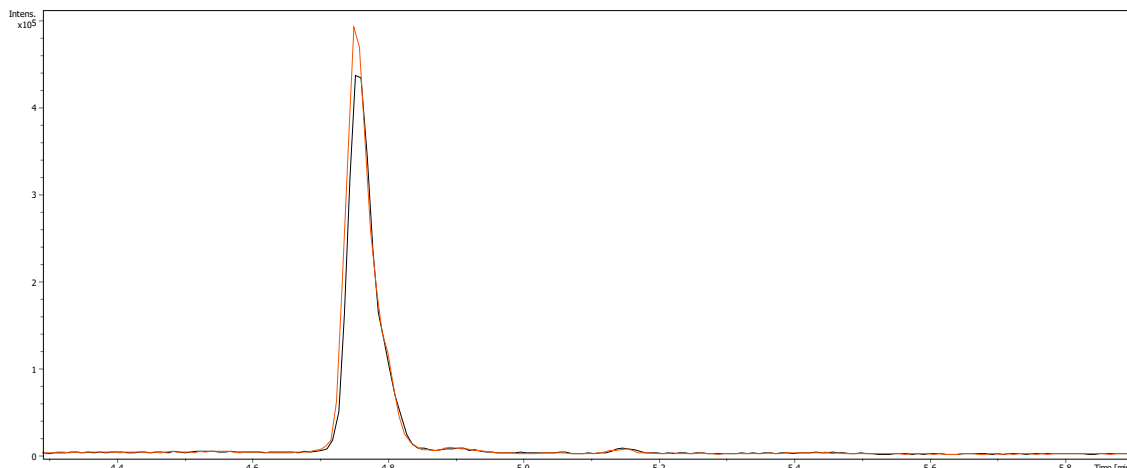
Obrázek 13 Porovnání vlivu přidavku 0,1% kyseliny mravenčí na intenzitu změřeného píku JH III (5 pmol). Vyšší intenzita zaznamenána u čistého 90% AcN (červená barva). Černou barvou je znázorněn pík pro JH III rozpuštěný v 90% AcN + 0,1% FA.
