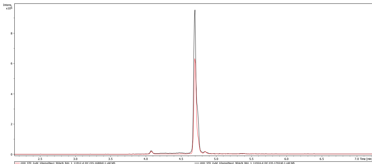
Obrázek 11 Kolona Astra C 8 . Překrývající se chromatogramy. Nástřik JH III byl 10 pmol. Červeně MF1(0,5% FA) - plocha píku 1478777, a černě MF2 ( 10 \mu\text{mol.l}^{-1} AmFA + 0,1 % FA) - plocha píku 2637262.
