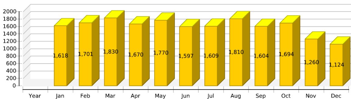
Obr. 7.1: Simulace solárních zisků [Polysun]
