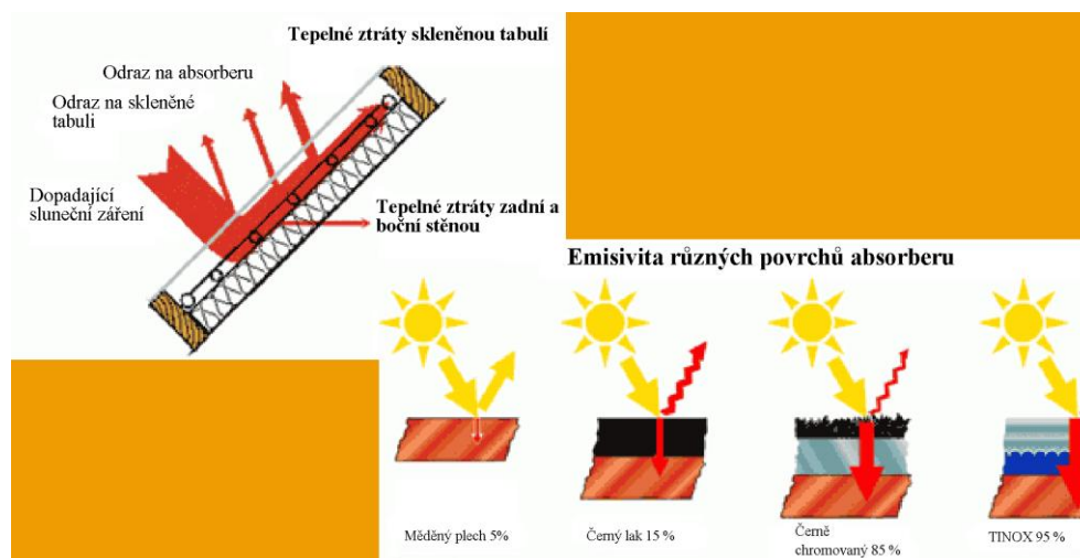
Obr. 2.7: Tepelné ztráty v solárním kolektoru [7]
