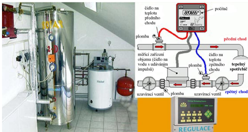
Obr. 2.12: Regulace solárního systému [7]
