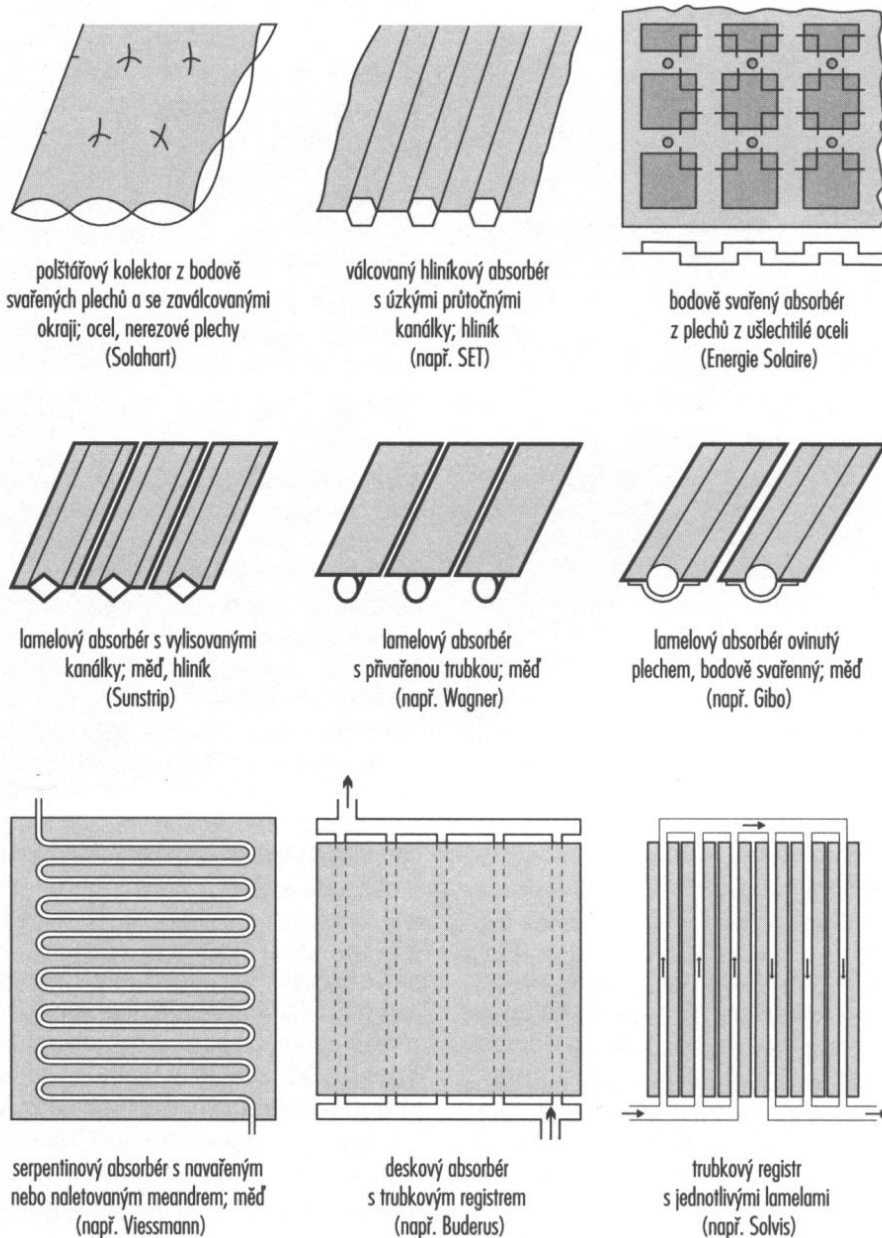
Obr. 2.9: Materiály a konstrukční formy absorberů [4]
