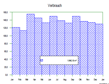
Bild 5: Jahresprofil für den Warmwasserverbrauch im Jugendheim, entwickelt aus den Messwerten und den Angaben des Haustechnikers
