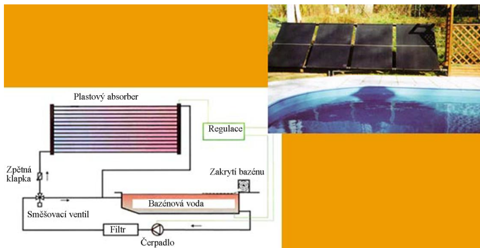
Obr. 2.3: Schéma ohřevu bazénové vody [7]
