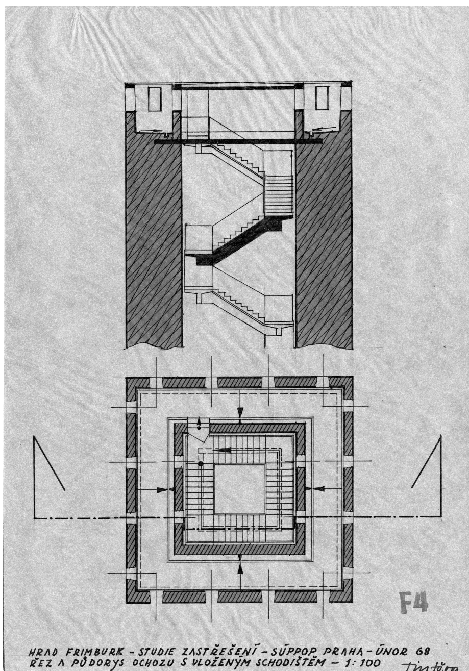
Obr. 5 Studie SÚPPOP v Praze na zastřešení věže z roku 1968
