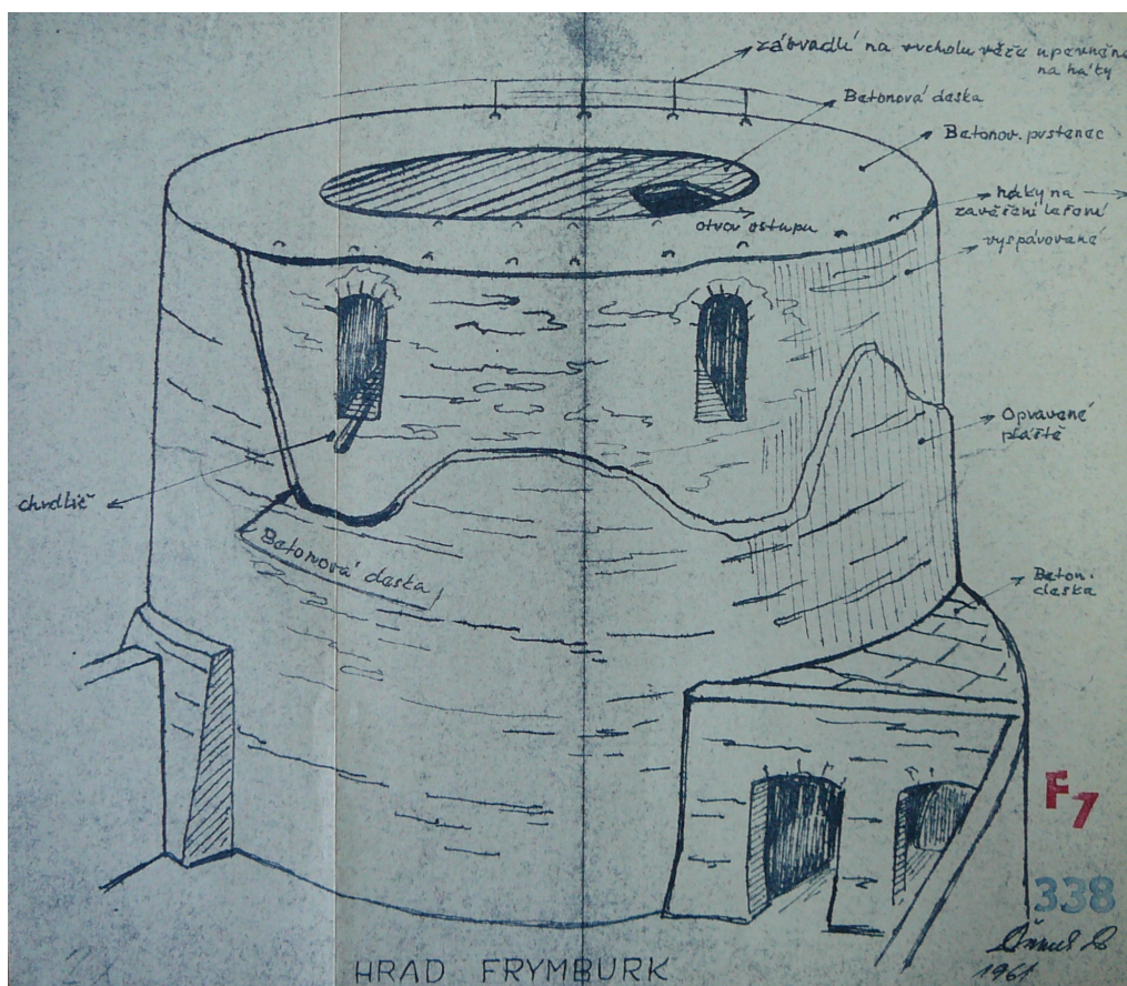
Obr. 2 Návrh Roberta Řemínka na úpravu věže z roku 1961
