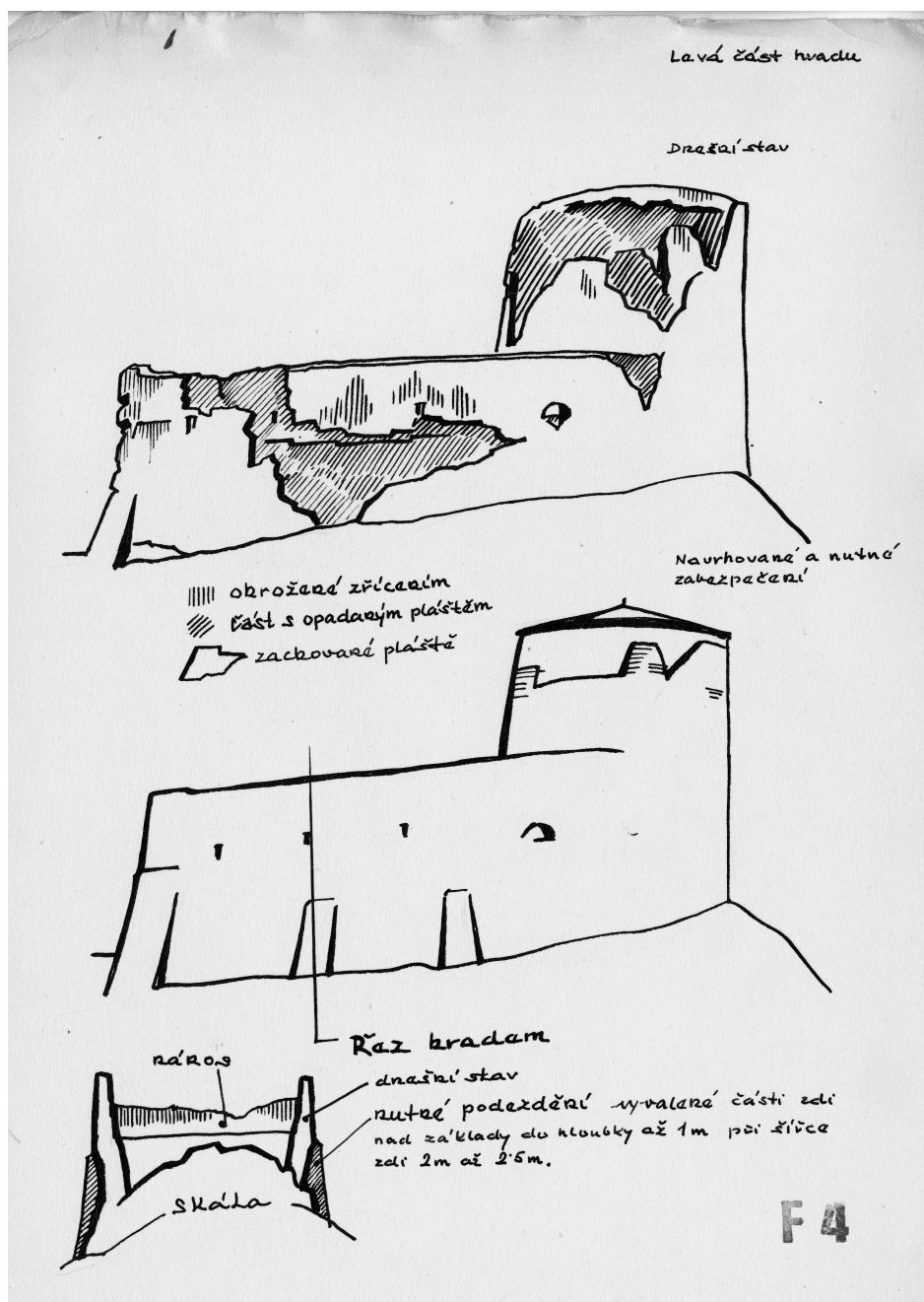
Obr. 4 Studie SÚPPOP v Praze na zabezpečení hradu z roku 1968
