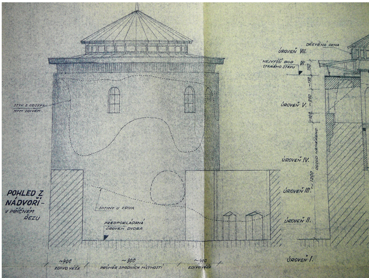
Obr. 8 Návrh Františka Novotného na úpravu věže z roku 1982
