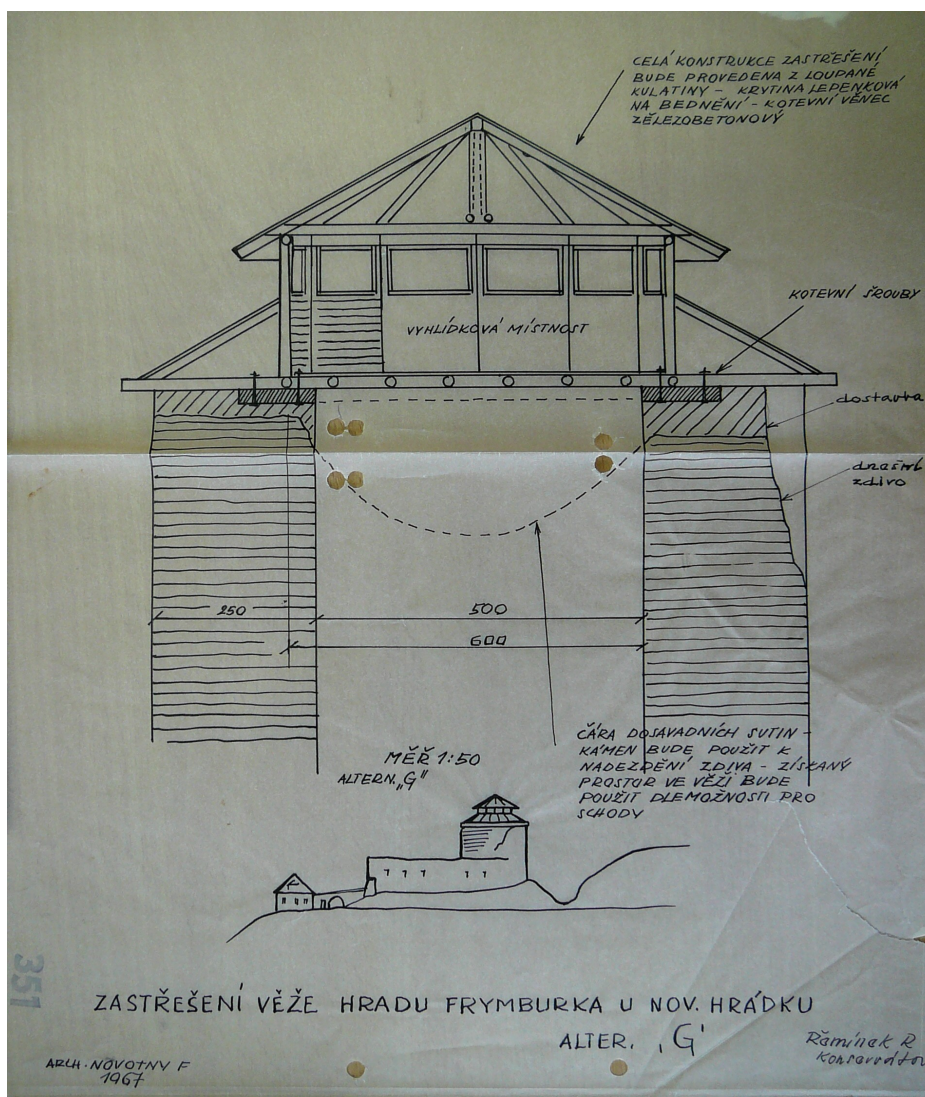
Obr. 3 Návrh Františka Novotného na zastřešení věže z roku 1967
