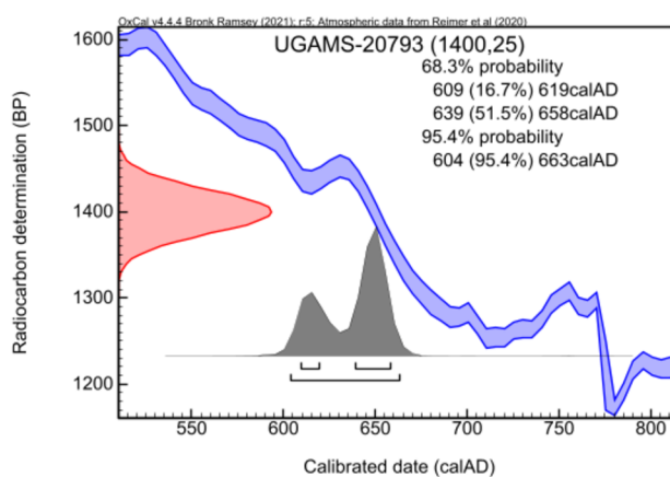
Obr. 13: kalibrace ^{14}\text{C} datace báze pylového profilu PALM13
