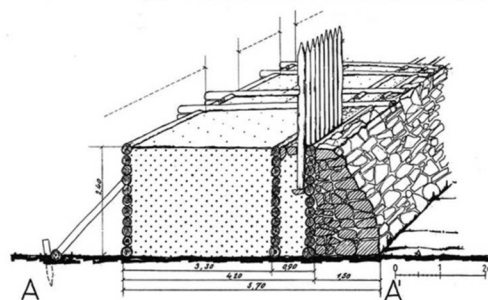
Obr. 3: Příklad úpravy komorové hradby s čelní kamennou plentou Kos (2012)
