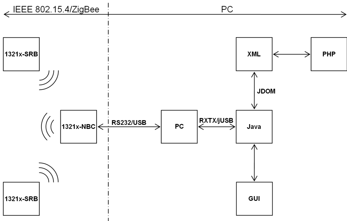
Obr. 3.6 Architektura bezdrátového hlasovacího zařízení.
