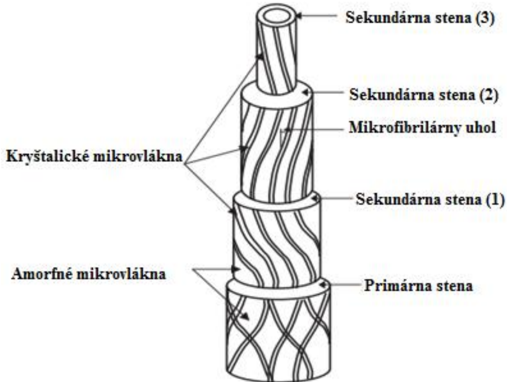
Obrázok 3 Štruktúra prírodných vlákien [19]
