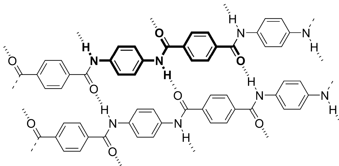
Obrázok 2 Znárodnenie vnútromolekulových väzieb v aramidoch [11]
