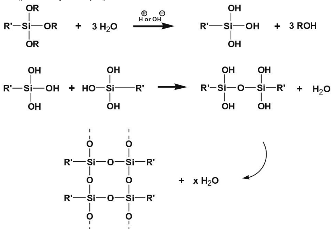
Obrázok 5 Hydrolýza a kondenzácia silanu [22]
