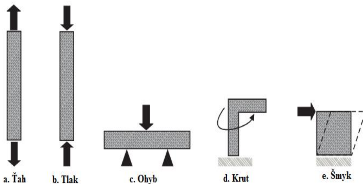
Obrázok 7 Typy síl [27]
