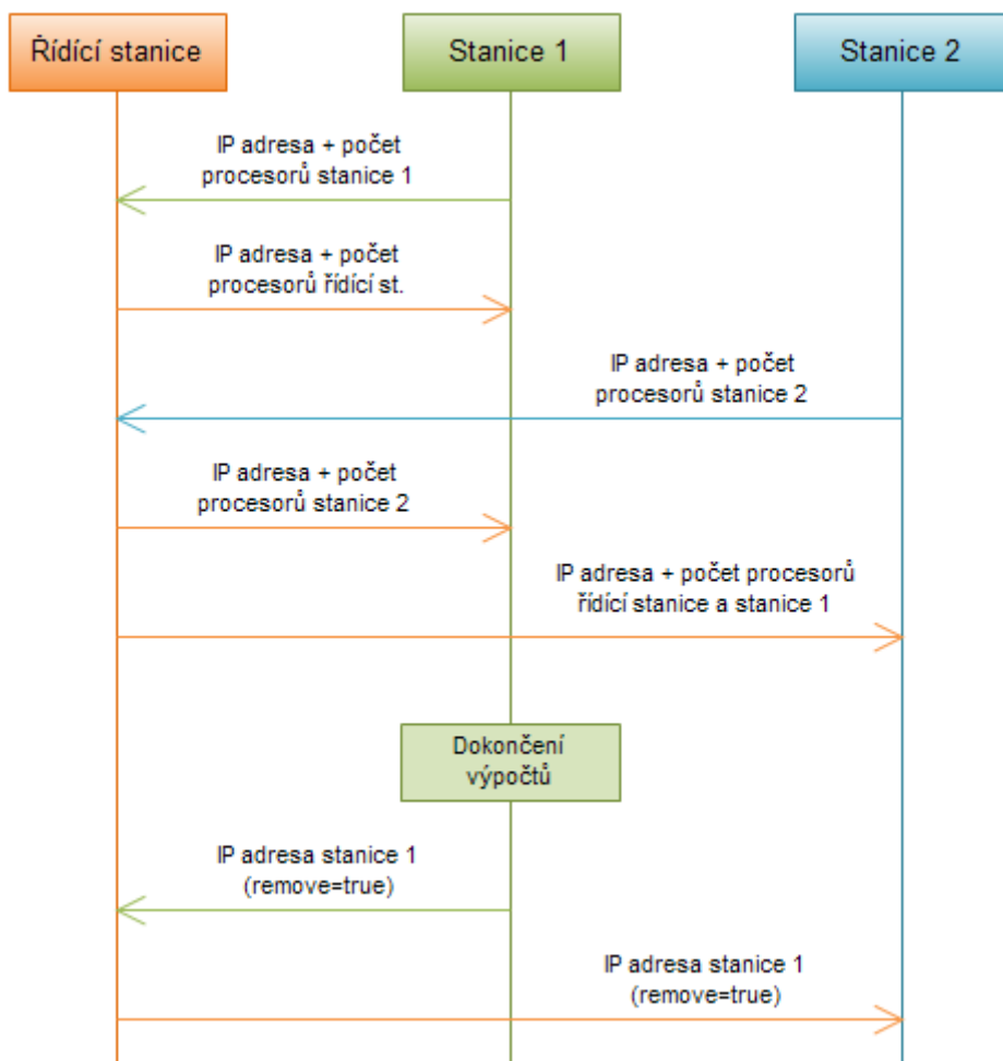
Obr. 2.3: Příklad komunikace mezi řídicí stanicí a odstaními stanicemi
