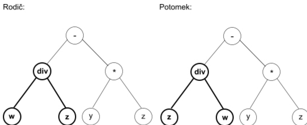
Obr. 1.5: Příklad operace permutace
