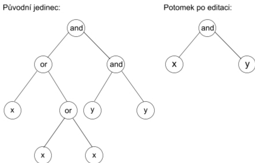
Obr. 1.6: Příklad operace editace
