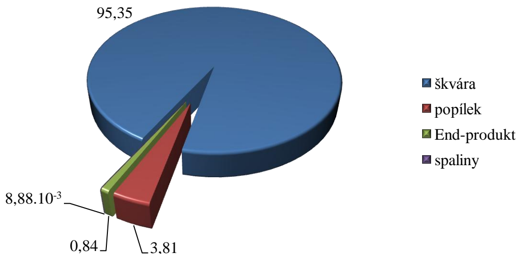
Obr. č. 45 Redistribuce Fe vztažená k produkovanému množství jednotlivých zbytků spalování [% hm.]
