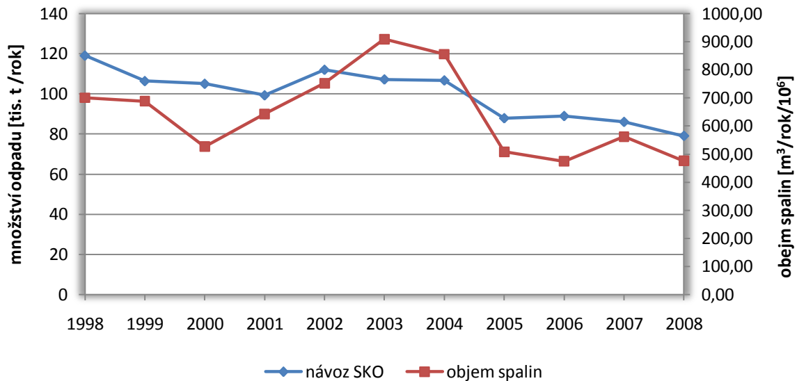
Obr. č. 46 Množství odpadu navezeného do spalovny a produkce spalin v letech 1998-2008 [34]
