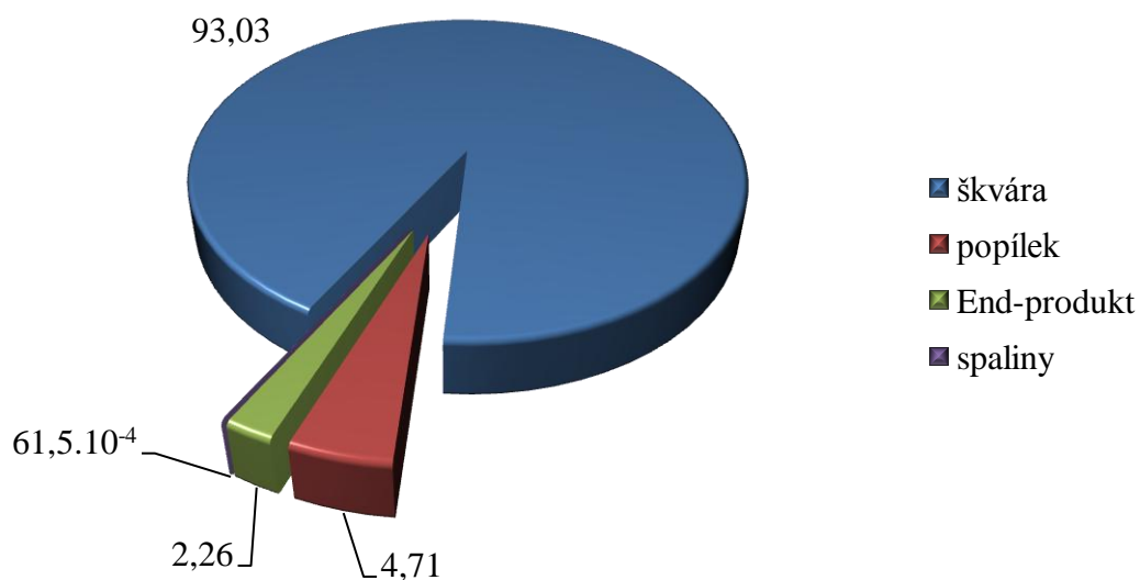
Obr. č. 34 Redistribuce Pb vztažená k produkovanému množství jednotlivých zbytků spalování [% hm.]
