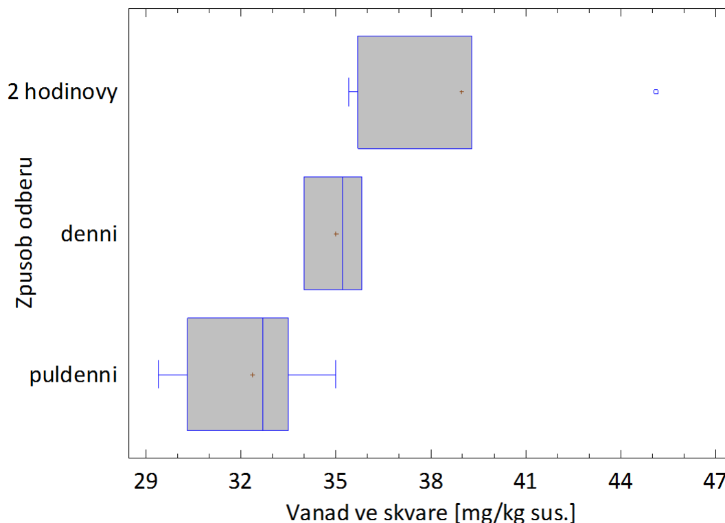
Obr. č. 39 Krabicový graf (Box and whisker plot)
