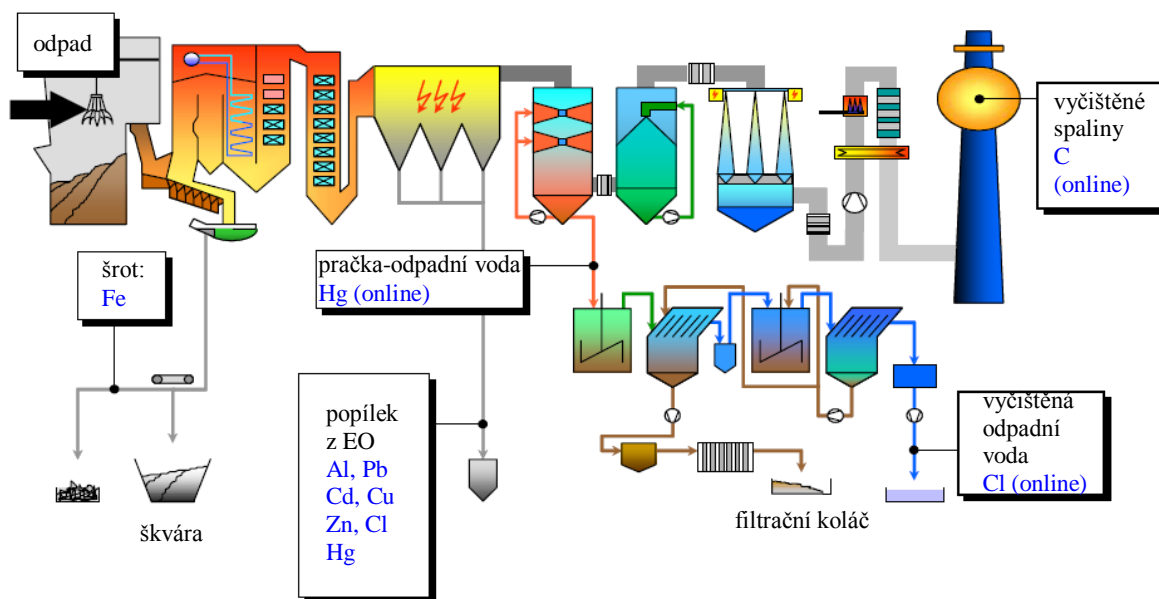
Obr. č. 8 Znárodnění procesu spalování, čištění spalin a měřících míst (MVA Spittelau)
