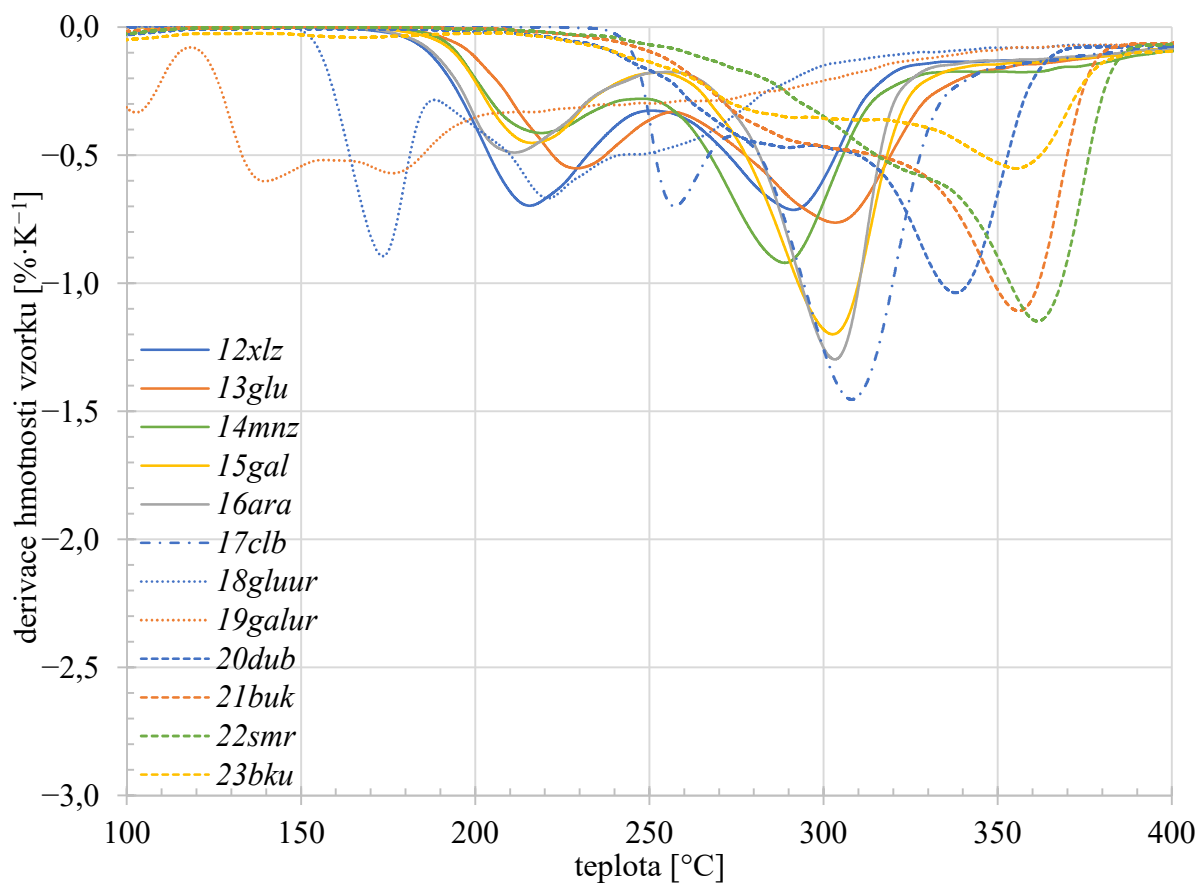
Obrázek 9.3. Derivace úbytku hmotnosti vzorků 1cel–11lig (nahore) a 12xlz–23bku (dole) při pyrolýze a rychlosti ohřevu 10 \text{ K} \cdot \text{min}^{-1} .
