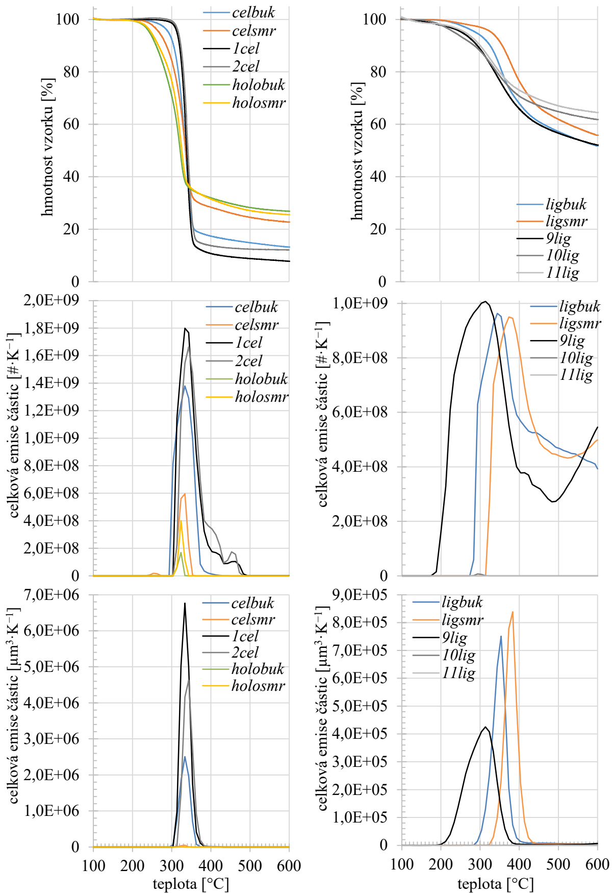
Obrázek 10.1. Průběh úbytku hmotnosti (nahore), početní (uprostřed) a objemové (dole) emise vzorků celulózy, hemicelulózy (vlevo) a ligninů (vpravo) při pyrolýze a rychlosti ohřevu 10 K·min -1 .
