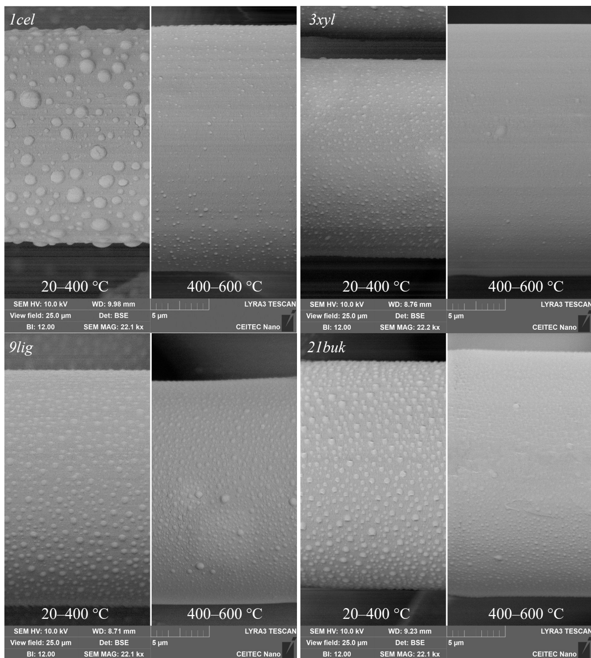
Obrázek 11.2. Rozdíl ve velikosti částic produkovaných při různých teplotách pyrolýzou Icel , 3xyl , 9lig a 21buk při rychlosti ohřevu 10 \text{ K} \cdot \text{min}^{-1} .
