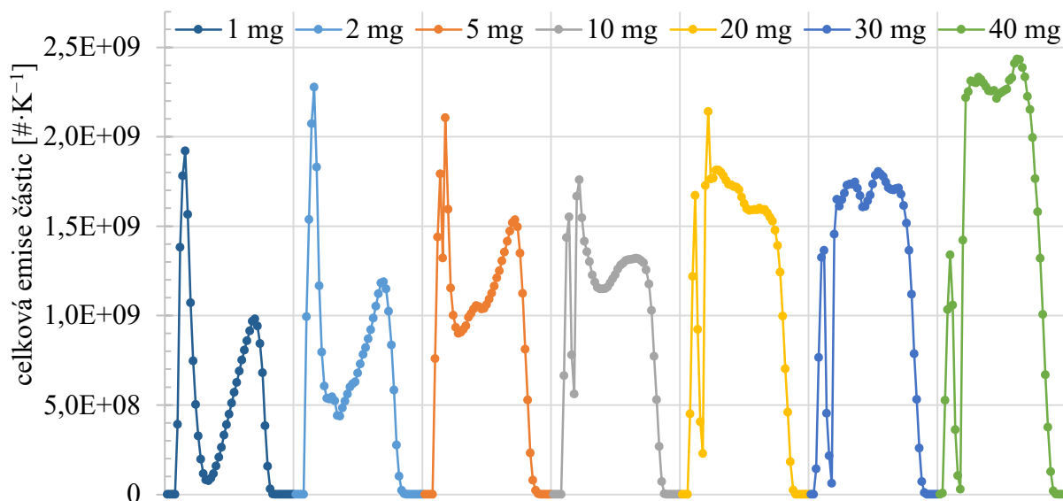
Obrázek 8.1. Celková emise částic při pyrolýze Icel pro různé hmotnosti vzorku.
