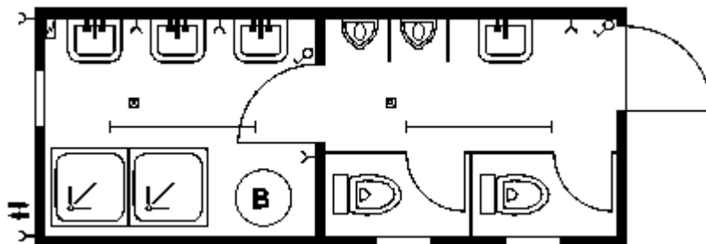
Obr. 5.16 – Sanitární kontejner Contimade Standart typ 19
