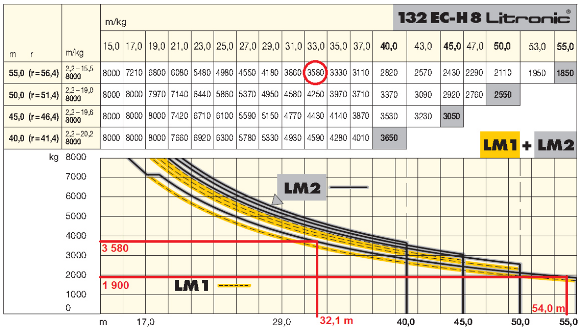
Obr. 6.6 – Zatěžovací křivka
