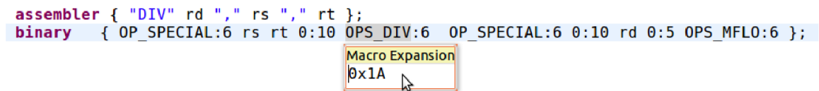
Obrázek 7.12: Ukázka makra v jazyce CodAL
