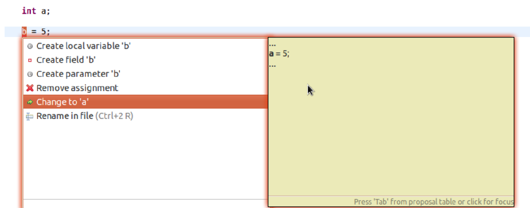
Obrázek 3.6: Seznam doporučení pro opravu sémantické chyby
