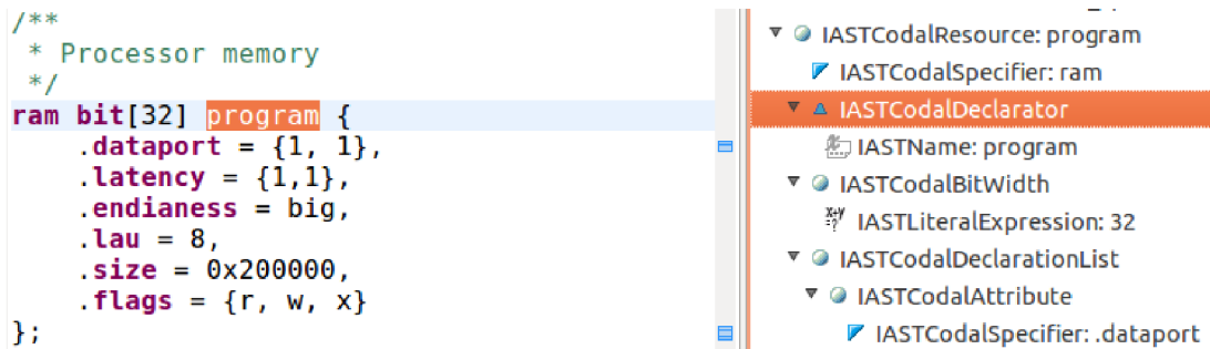
Obrázek 7.2: Ukázka použití pohledu DOM AST Viewer
