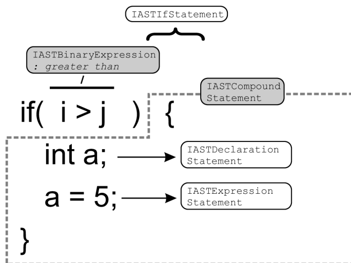
Obrázek 7.5: Příklad interpretace příkazu v AST
