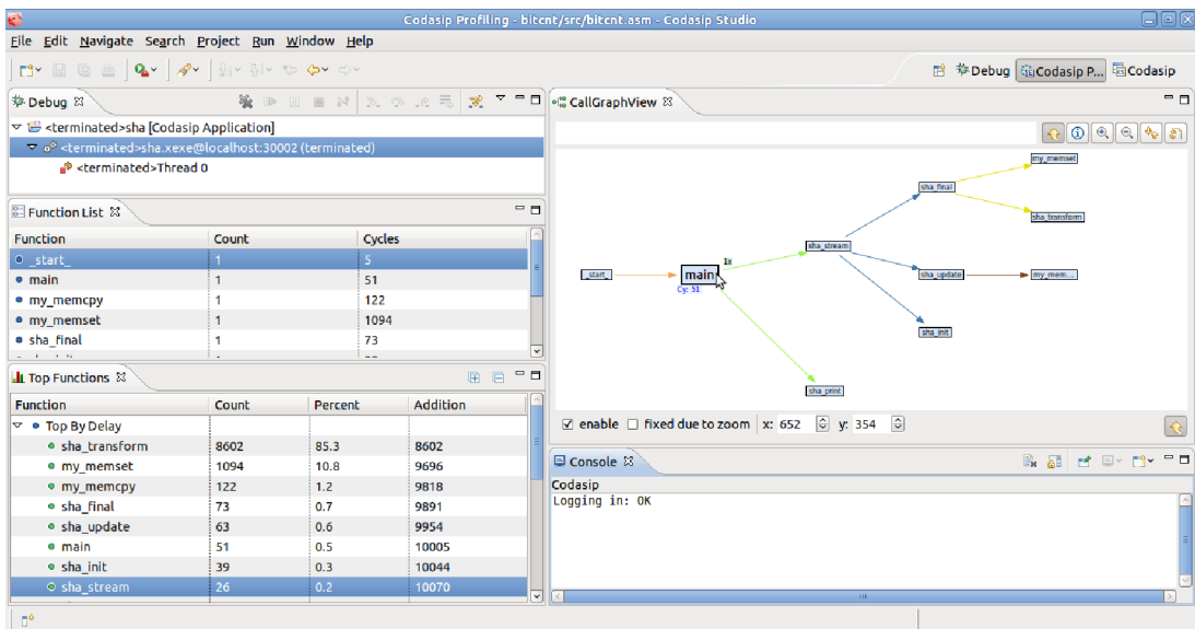
Obrázek 1.1: Profilování pomocí nástroje Codosip Studio
