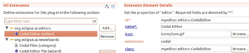
Obrázek 3.10: Karta deklarace editoru v souboru plugin.xml
