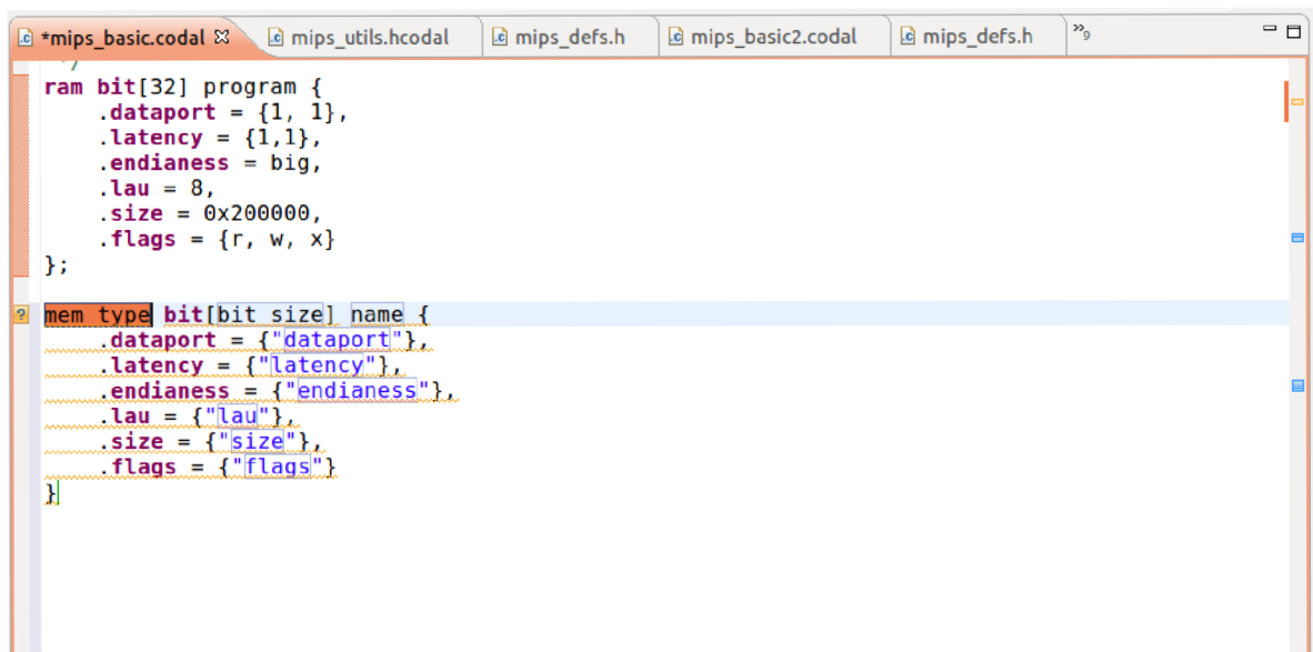
Obrázek A.8: Vložení šablony do zdrojového kódu
