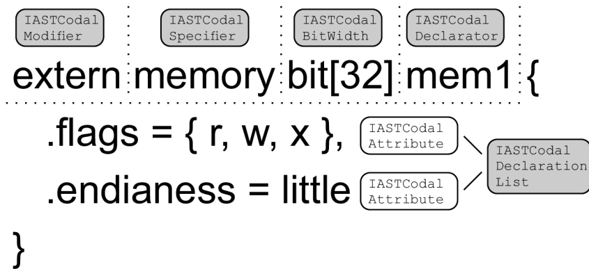
Obrázek 7.9: Příklad interpretace zdrojů v AST
