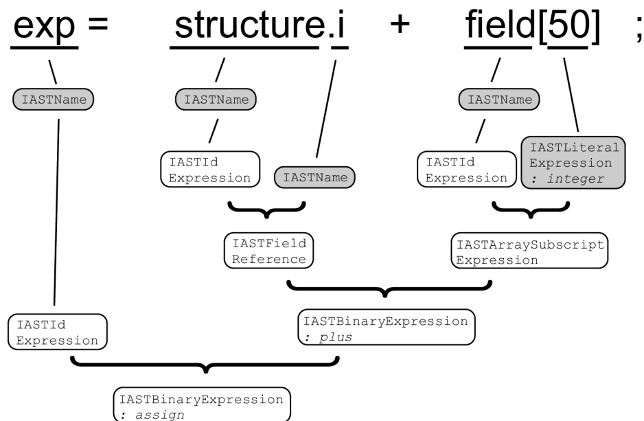
Obrázek 7.4: Příklad interpretace výrazu v AST
