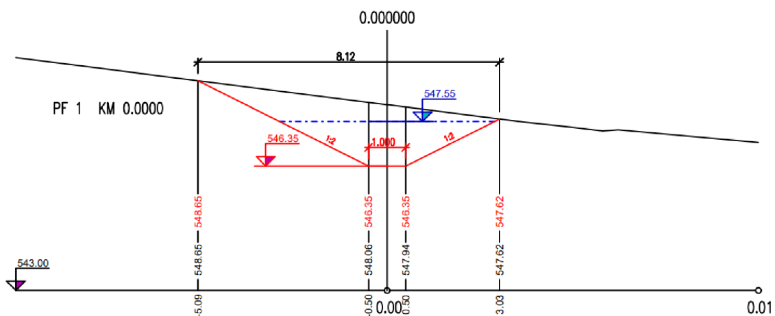
Obr. 45 ZP6 – Priečný rez – bez hrádky
