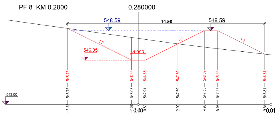
Obr. 46 ZP6 – Priečný rez – s hrádkou
