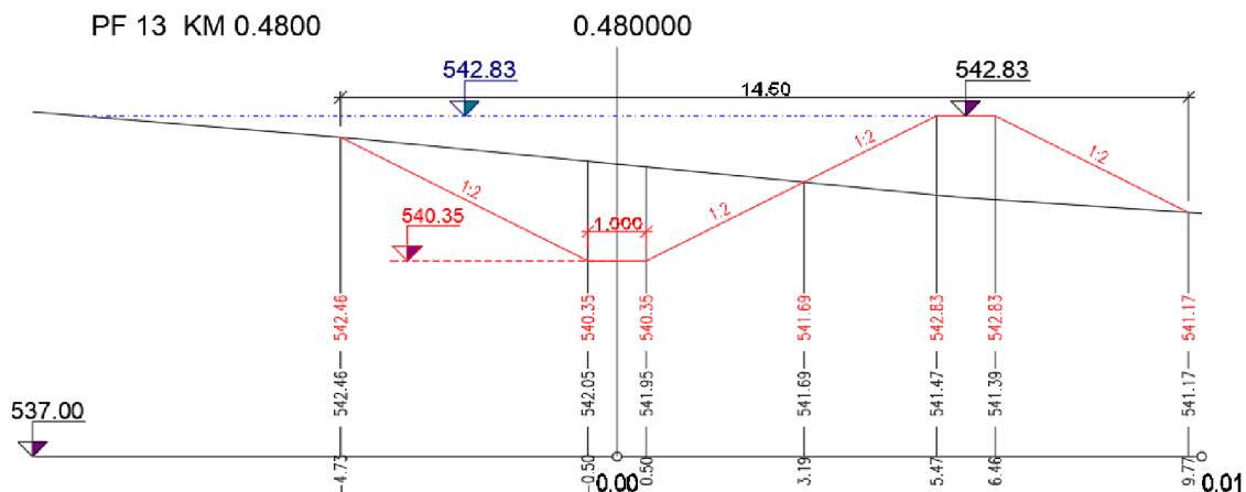
Obr. 42 ZP4 – Pričný rez – s hrádzkou
