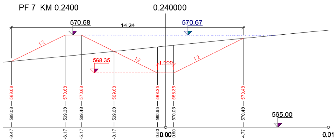
Obr. 40 ZP3 – Priečný rez – s hrádkou
