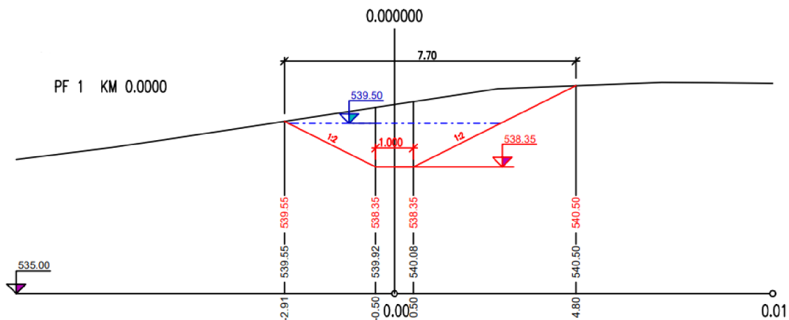
Obr. 49 ZP8 – Priechý rez – bez hrádzky
