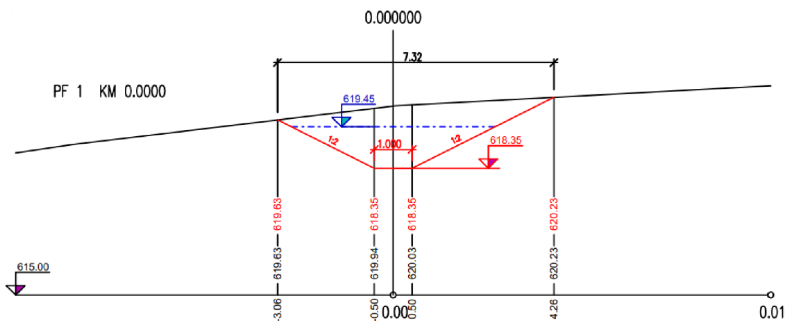
Obr. 53 ZP10 – Priečny rez – bez hrádzky
