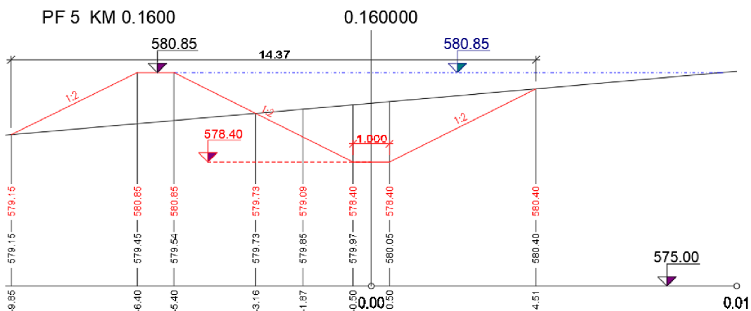
Obr. 38 ZP2 – Priečný rez – s hrádzkou
