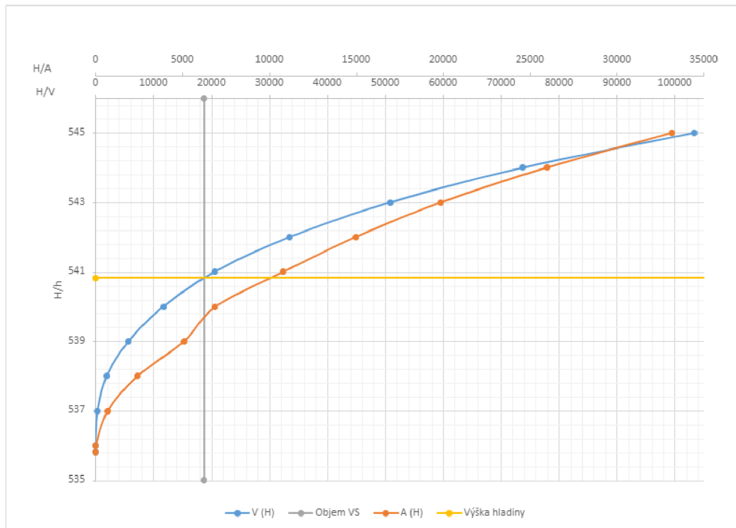
Obr. 61 Graf – Batygrafické krivky ON1
