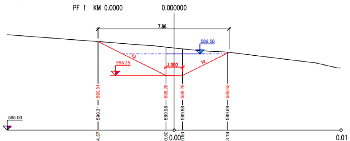
Obr. 35 ZP1 – Priečný rez – bez hrádzky
