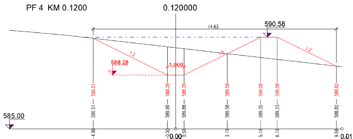
Obr. 36 ZP1 – Priechny rez – s hrádkou
