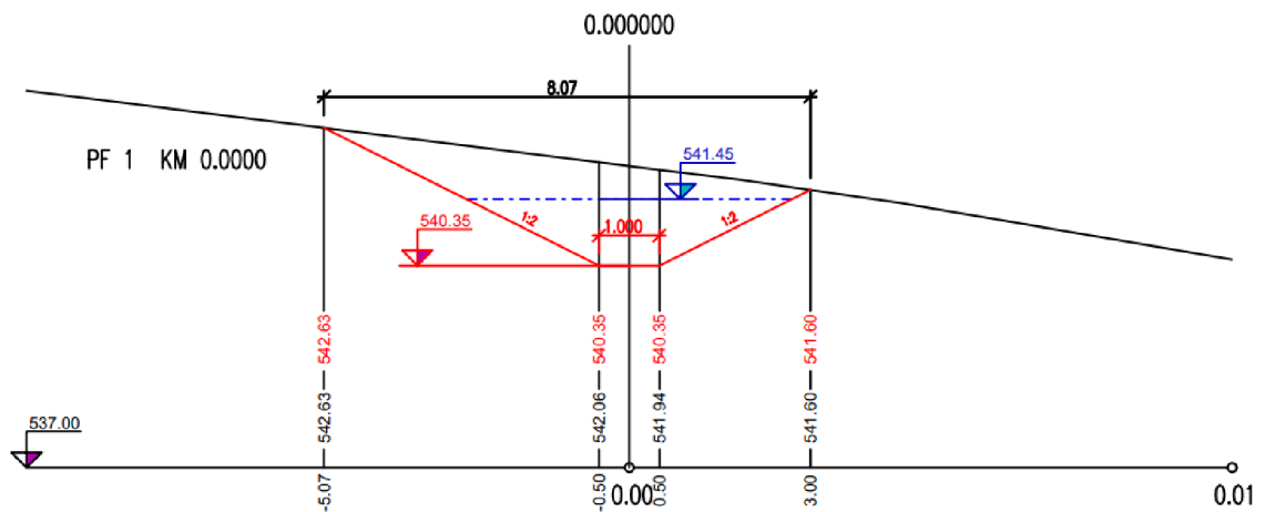
Obr. 43 ZP5 – Priechny rez – bez hrádzky
