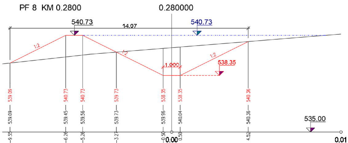
Obr. 50 ZP8 – Priechý rez – s hrádzkou
