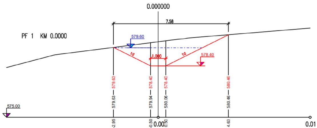
Obr. 37 ZP2 – Priečný rez – bez hrádzky
