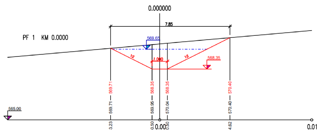
Obr. 39 ZP3 – Priečný rez – bez hrádky
