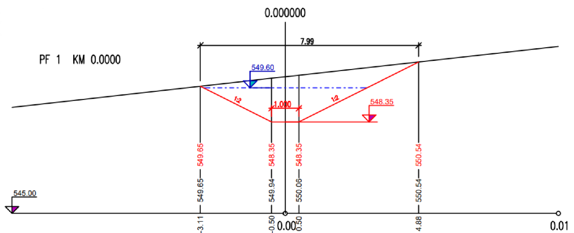
Obr. 47 ZP7 – Priečný rez – bez hrádzky
