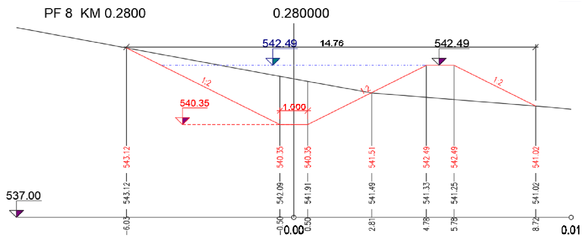
Obr. 44 ZP5 – Priechny rez – s hrádzkou
