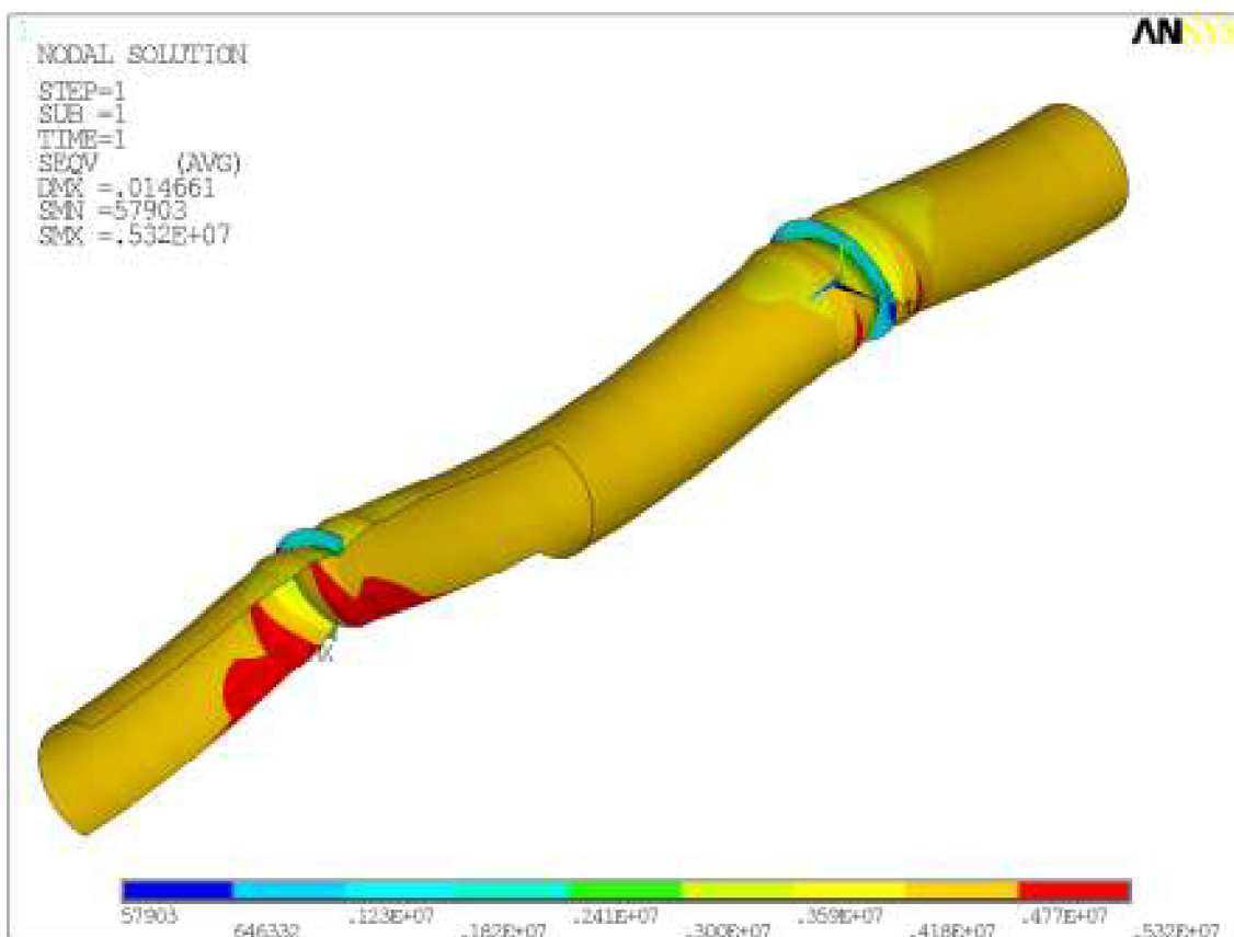
Obr. 5.29 Misesovo napětí od vlastní tíhy a přetlaku (kombinace K1)
