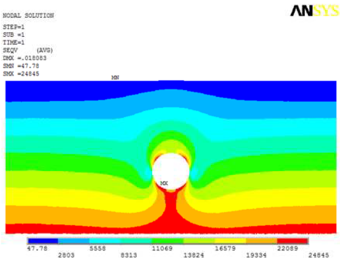
Obr. 5.15 Průběh Misesova napětí v zemině pro boční vzdálenost 4d
