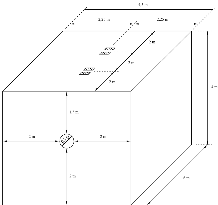
Obr. 5.19 Základní geometrie prostorového modelu
