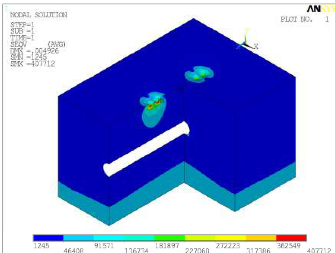
Obr. 5.23 Průběh napětí
