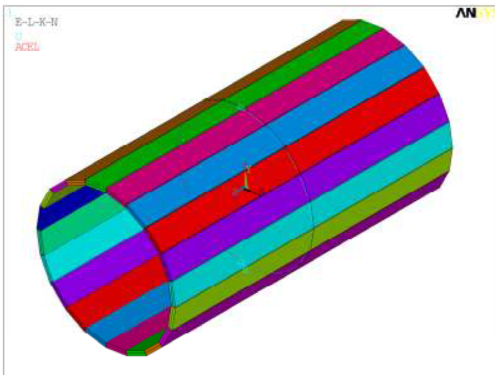
Obr. 5.3 Model z prutových prvků BEAM 44 (se zapnutým vykreslením tvaru)
