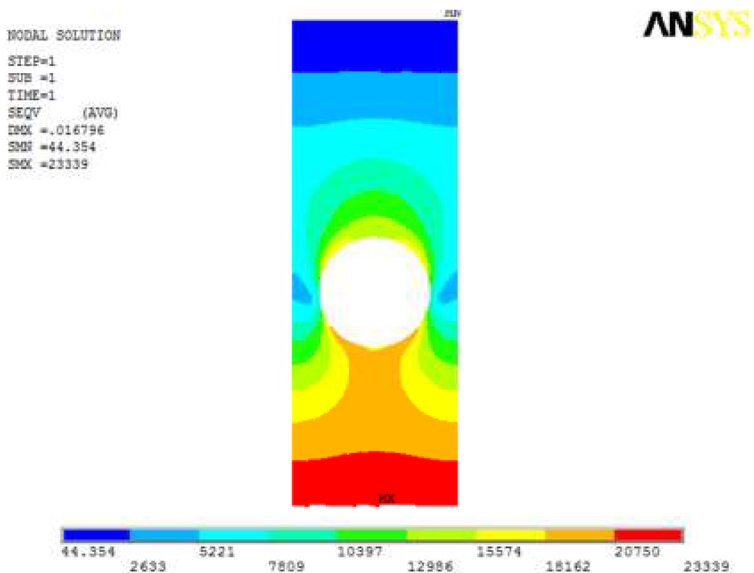
Obr. 5.14 Průběh Misesova napětí v zemině pro boční vzdálenost 0,25d
