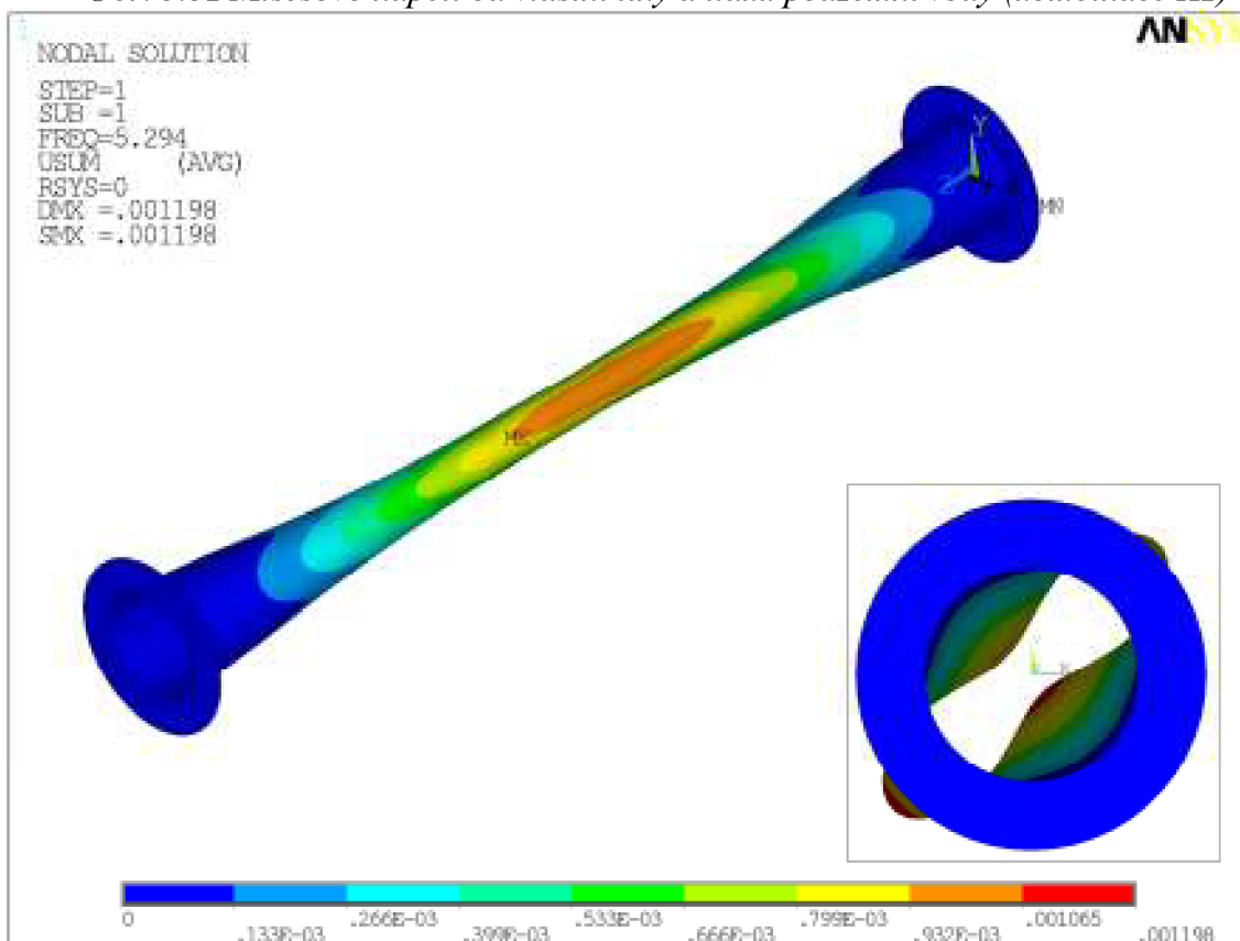
Obr. 5.33 První vlastní tvar ( \lambda_1 = 5,294 ) od vlastní tíhy a tlaku podzemní vody (kombinace K2)
