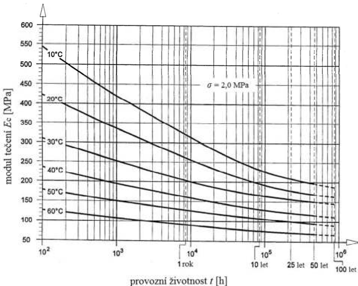
Obr. 3.2 Moduly tečení vysokohustotního polyethylenu PE100 [19]
