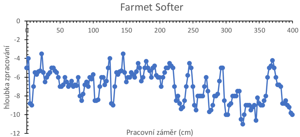
Graf 5 Zpracování profilu dna strojem Farmet Softer
