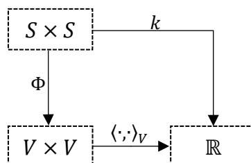
graf. 5.1.a – platí pro jádro k , Hilbertův prostor V a zobrazení \Phi .
