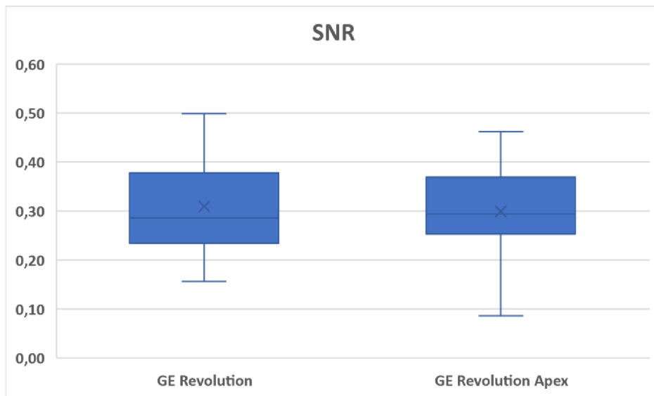
Obrázek 21 Graf pro porovnání hodnot SNR
