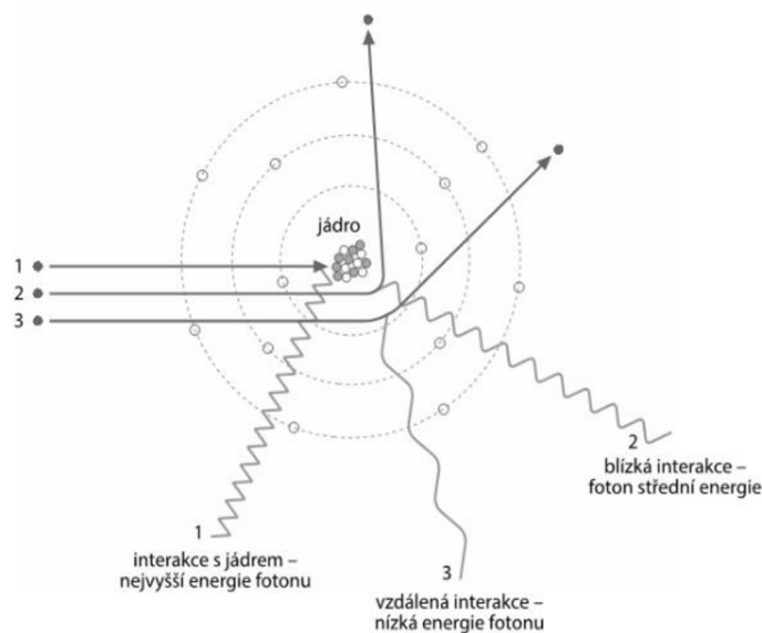
Obrázek 1 Interakce elektronů při vzniku brzdného záření
