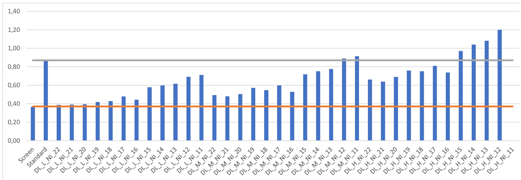
Obrázek 16 Graf NI a SNR
