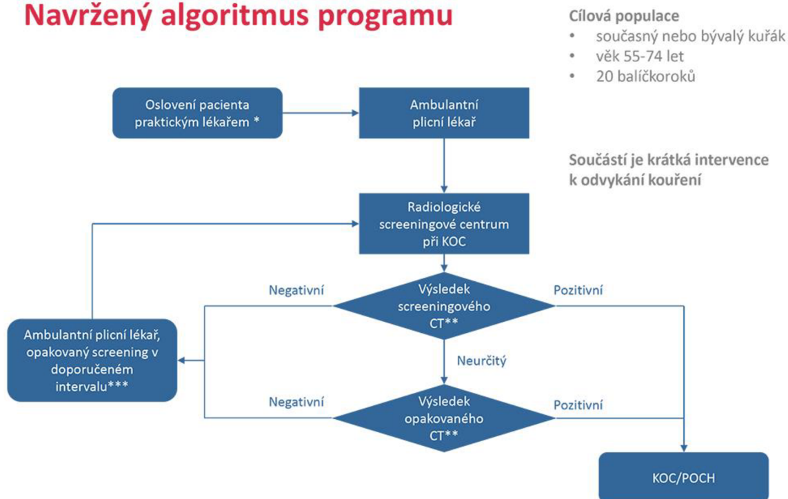
Obrázek 3 Algoritmus screeningového procesu
