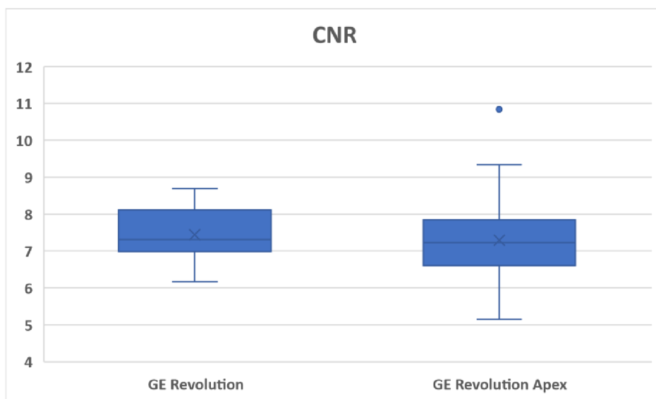
Obrázek 22 Graf pro porovnání hodnot CNR
