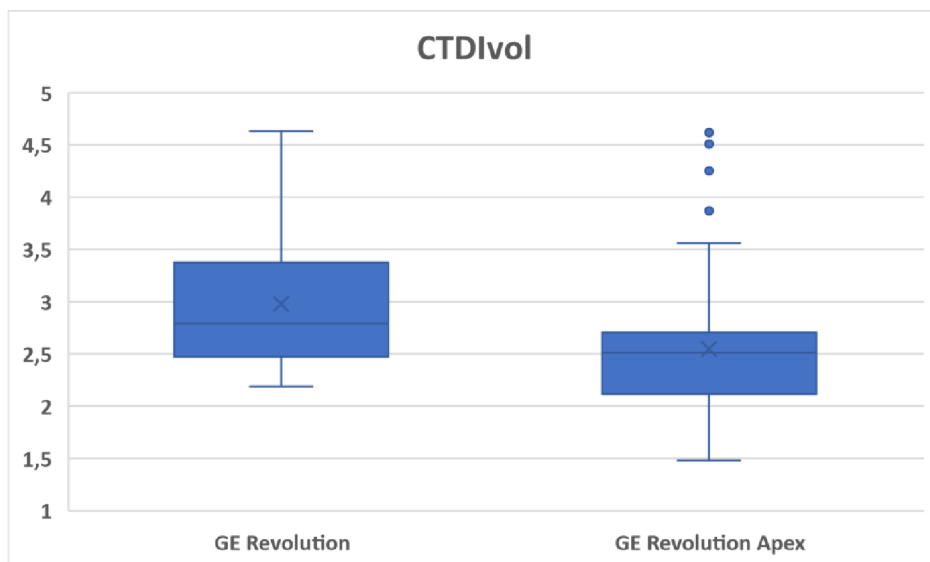
Obrázek 19 Graf pro porovnání hodnot CTDIvol
