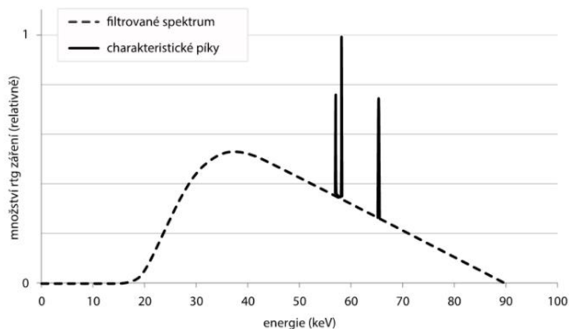
Obrázek 2 Rentgenové spektrum brzdné a charakteristické záření
