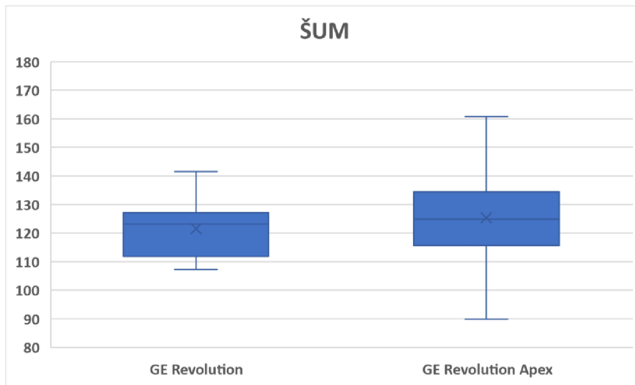
Obrázek 20 Graf pro porovnání hodnot šumu
