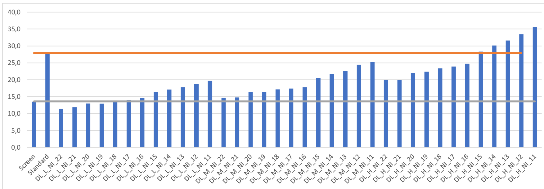
Obrázek 15 Graf NI a CNR
