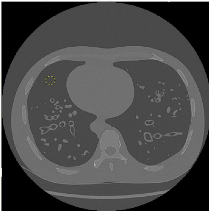
Obrázek 13 ROI v plicní tkáni
