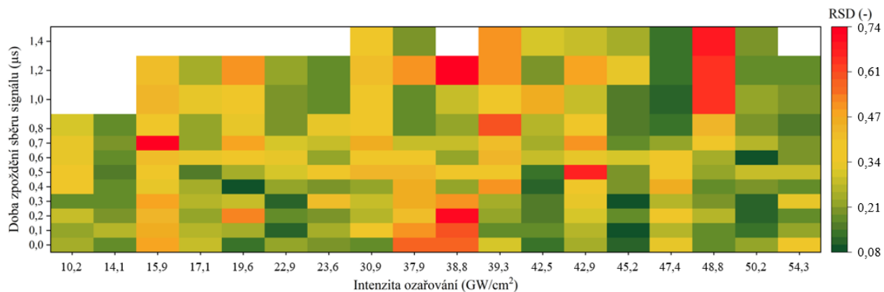
Obrázek 21: Závislost relativní směrodatné odchylky (RSD) SNR na intenzitě ozařování a době zpoždění sběru signálu pro vlnovou délku 1064 nm za laboratorních podmínek zobrazena pomocí teplotní mapy.
