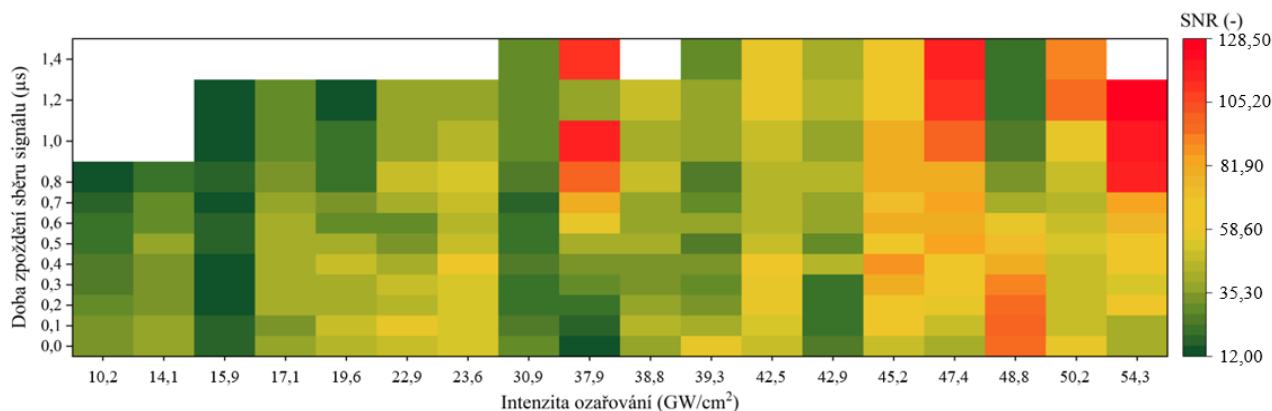
Obrázek 20: Závislost SNR na intenzitě ozařování a době zpoždění sběru signálu pro vlnovou délku 1064 nm za laboratorních podmínek zobrazena pomocí teplotní mapy.
