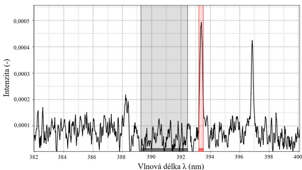
Obrázek 9: Příklad získaného spektra pro analýzu SNR – červená oblast znázorňuje spektrální čáru analyzovaného prvku (signál) a černá oblast tzv. noise (šum).
