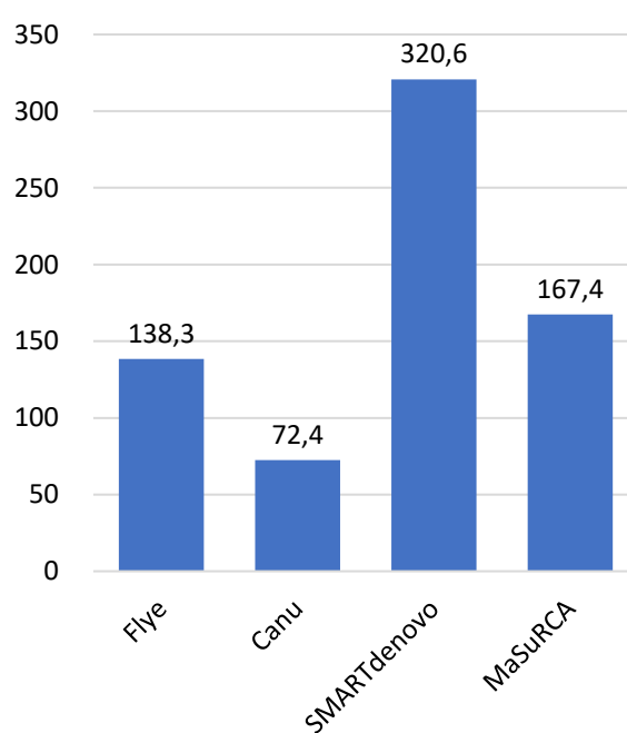
Obrázek 14: Výsledky nástroje BioKit pro Flye, Canu, SMARTdenovo a MaSuRCA. A – Celková délka referenční sekvence v gigabázích, B – Počet kontigů, C – L50, D – N50 v kilobázích.
