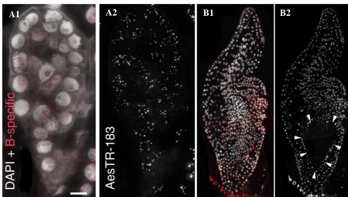
Obrázek 3: Fluorescenční in situ lokalizace B specifické sondy na řezech embryí A. speltoides . B-specifická sonda AesTR-183 je na sloučených obrázcích (A1, B1) znázorněna červeně . Na obrázcích A2, B2 je zdůrazněna pouze vrstva s B-specifickým signálem v bílém zobrazení. A – 5 DAP embryo s B chromozómem ve všech buňkách. Měřítko 10 \mu m. B – 15 DAP embryo, šipky ukazují na region kořene bez přítomnosti B chromozómů. Měřítko 100 \mu m. Modifikováno z Ruban et al., 2020.
