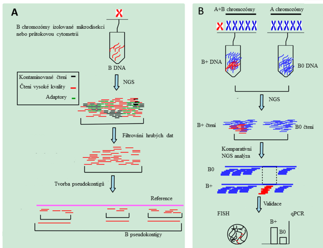
Obrázek 9: Metody studia sekvence B chromozómu. A – Přímá metoda. B chromozóm je izolován mikrodisekci nebo průtokovou cytometrií. Izolovaná DNA je sekvencována a přefiltrována hrubá data jsou bioinformatickými nástroji překrývána za tvorby pseudokontigů. B – Nepřímá metoda. DNA izolována z karyotypu s B chromozómy a DNA bez B chromozómů je sekvencována. Sekvence B chromozómu jsou získané komparativní analýzou NGS čtení obou datasetů. Modifikováno z Ahmad & Martins, 2019.
