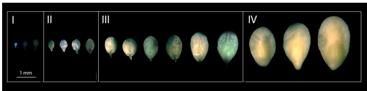
Obrázek 17: Vývojová řada embryí S. purpureosericeum . Členěno dle cílových skupin relevantních pro experimenty. 1. skupina – 7DAP, 2. skupina – 14DAP, 3. skupina – 21DAP, 4. skupina – 28 DAP. Měřítko 1 mm.
