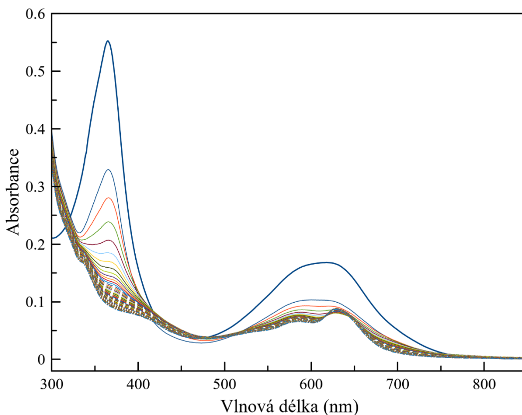
Obr. 12: Absorpční spektra fcb s ionty kobaltu v metanolu měřeny každé 2 min po dobu 2 hod. Modře je znázorněno spektrum volného fycocyanobilinu před přidáním kovu.
