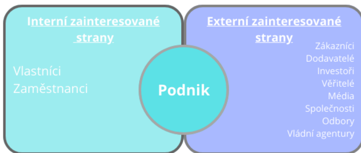
Obrázek 2: Klasifikace stakeholderů
