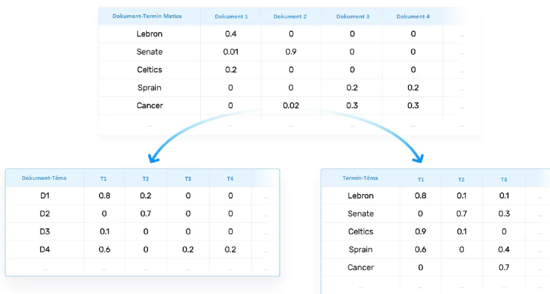
Obr. 1 Rozklad matice dokument-termín na matice dokument-téma a termín-téma. Zdroj: podle [15] upravil autor.
