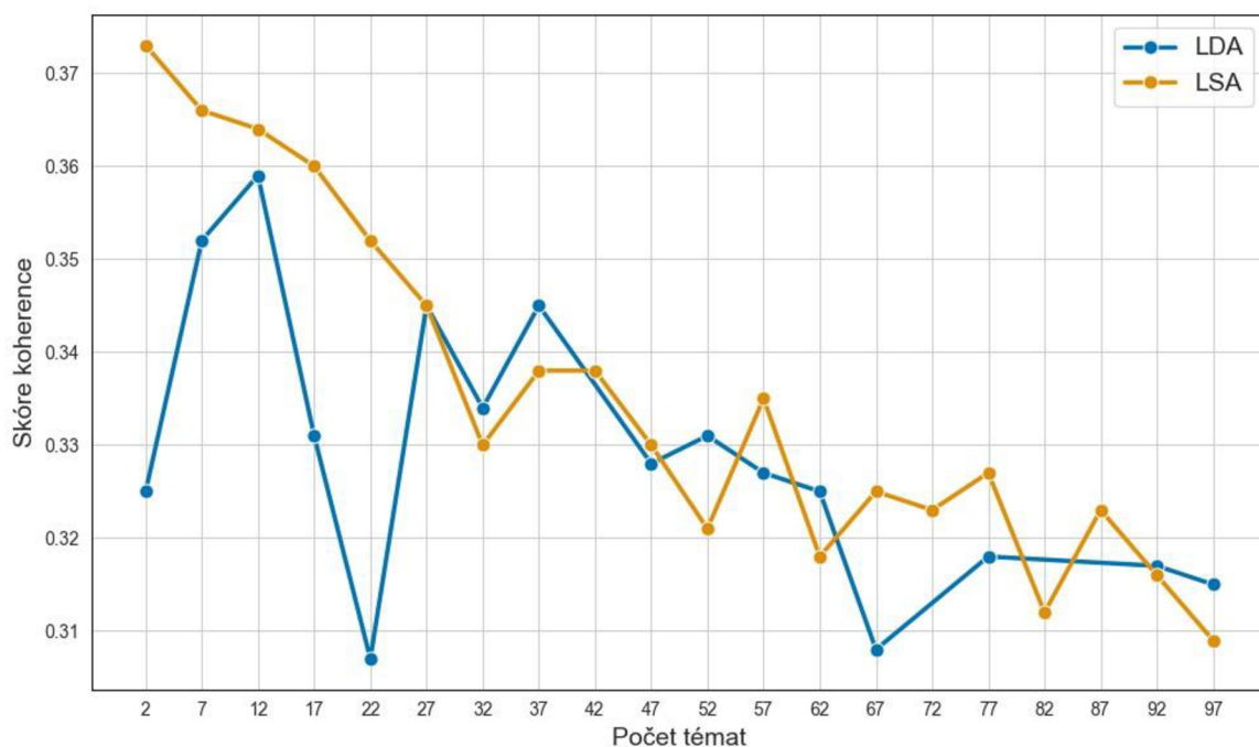
Obr. 15 Graf vývoje koherence Sklearn LDA a LSA modelů pro různé hodnoty počtu témat. Zdroj: Autor
