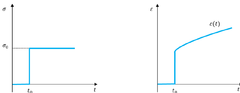
Obr. 3 Creep (Zhang, 2021)
