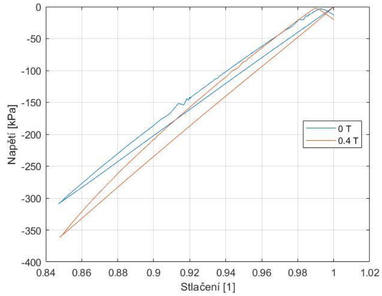
Obr. 33 Napětí při poloviční rychlosti zatěžování
