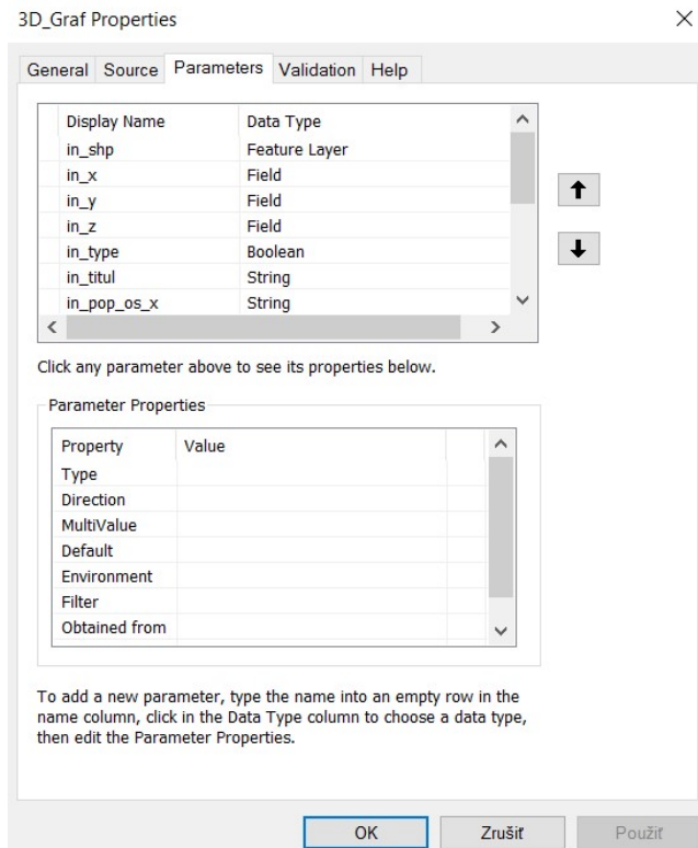
Obr. 34: Parametry skriptu v příkladu 3D Grafy
