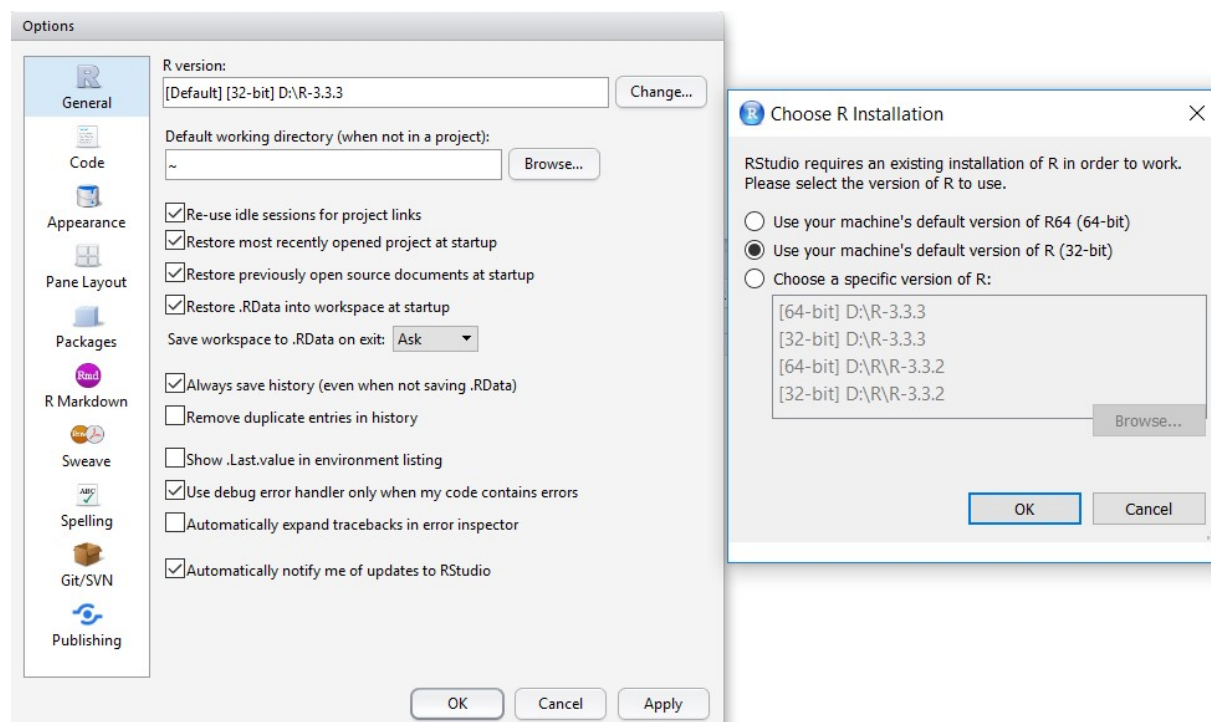
Obr. 64: Nastavení 32-bitové verze R Project
