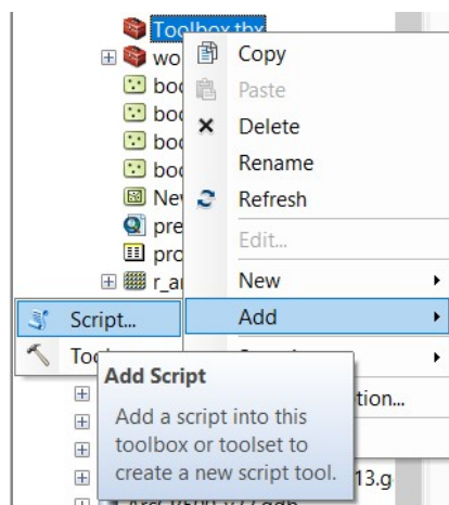
Obr. 68: Přidání skriptu
