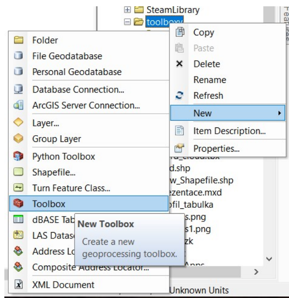
Obr. 67: Nový Toolbox
