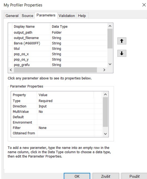
Obr. 23: Parametry skriptu v příkladu příčný profil
