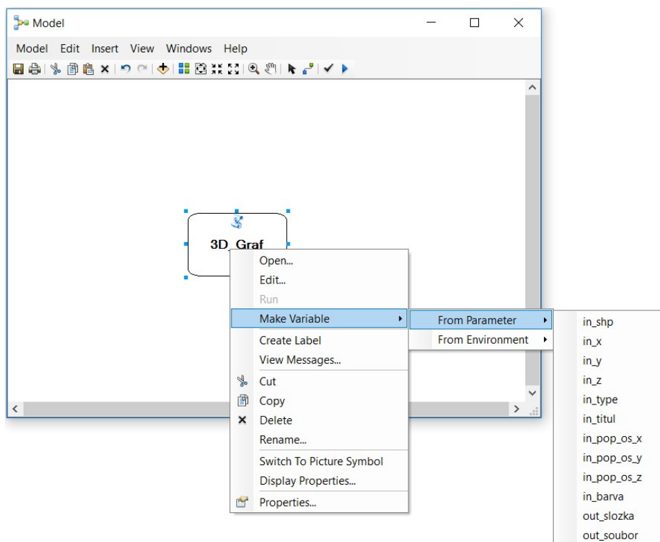
Obr. 36: Model příkladu 3D Grafy
