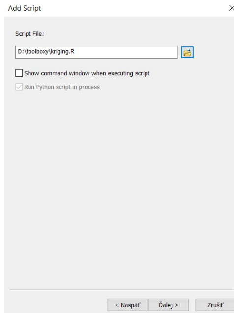
Obr. 70: Zadání R-Skriptu
