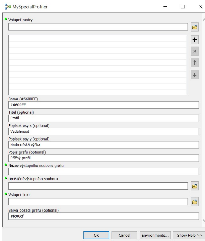
Obr. 72: Uživatelské rozhraní
