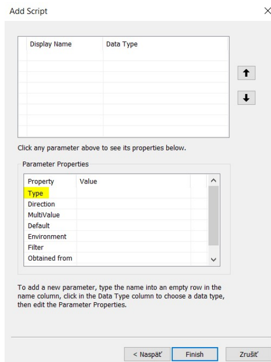
Obr. 71: Parametry skriptu
