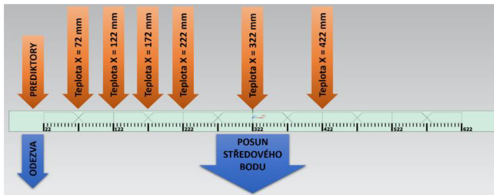
Obr. 9 Schéma prediktorů a odezvy pro odhad posunu středu stupnice
