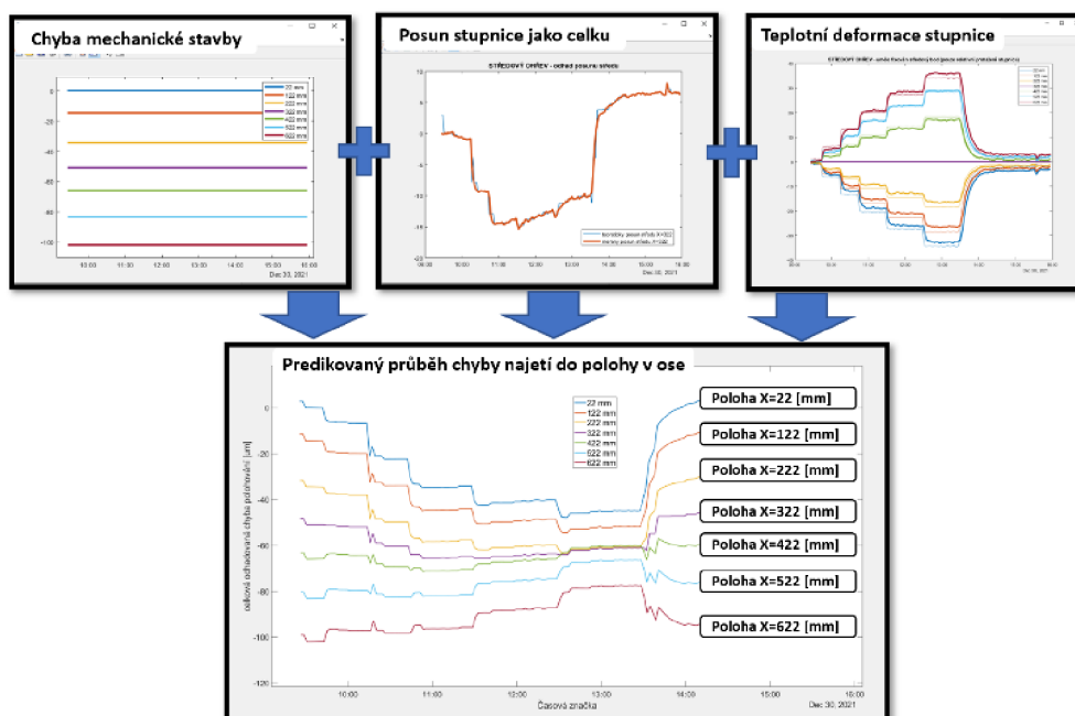
Obr. 10 Sloučení dílčích přírůstků chyby
