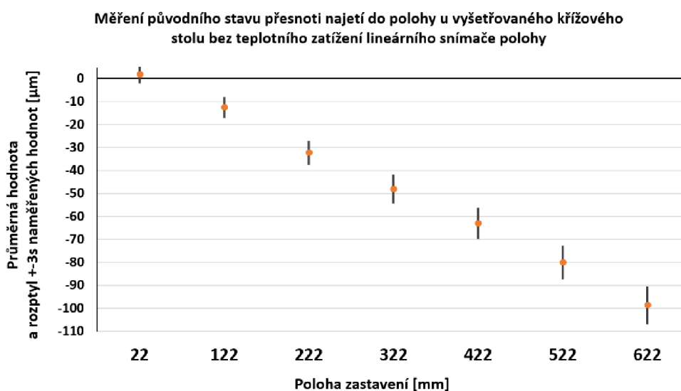
Obr. 7 Měření změny odchylky polohování vlivem změny okolního prostředí těžké laboratoře
