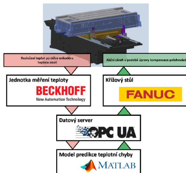
Obr. 6 Datová struktura zpětnovazební smyčky křížového stolu
