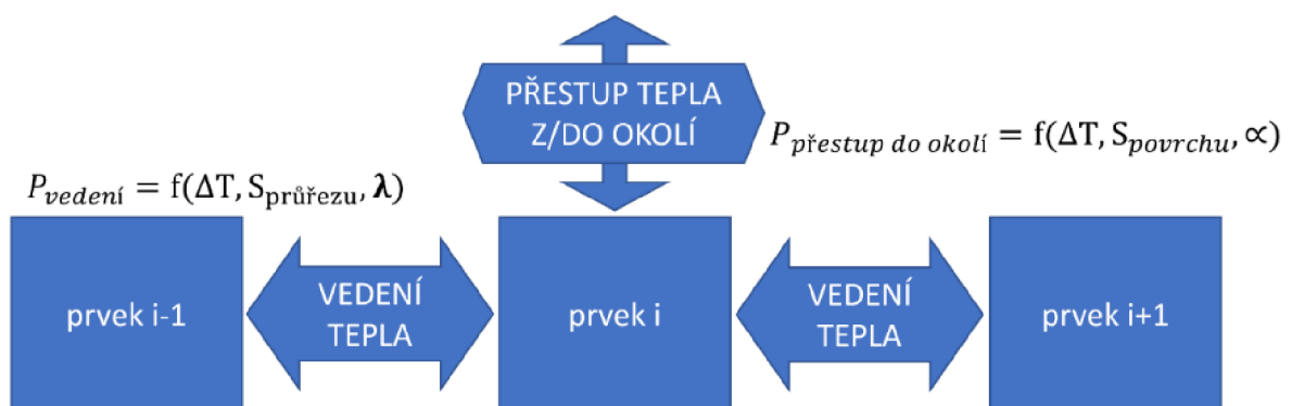
Obr. 8 Model 1D šíření tepla lineárním snímačem polohy
