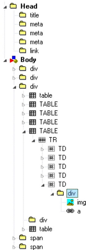
Obrázek 3.1: Typický strom tagů v HTML stránce
