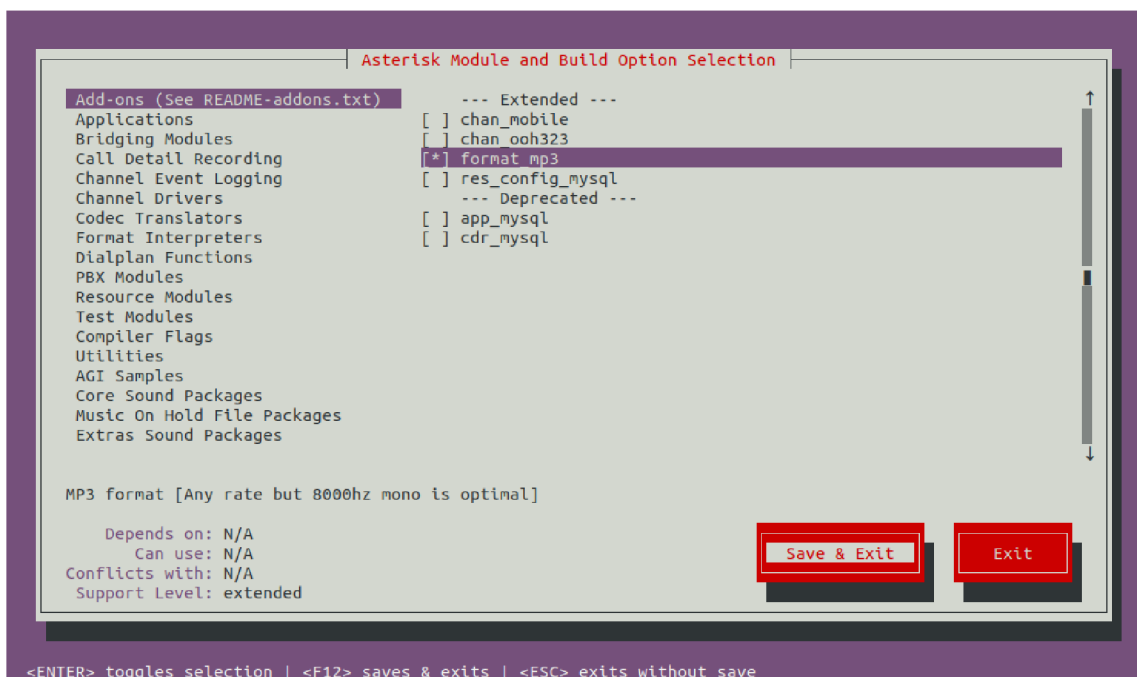
Obr. 3.6: Vybrání volitelných modulů pro Asterisk.
