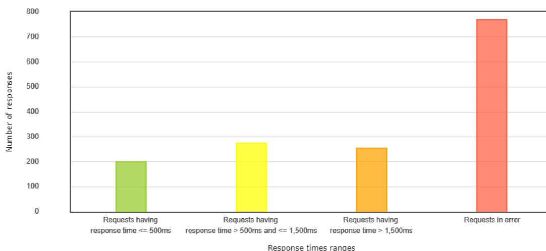
Obr. 3.17: Přehled odezvy ústředny při zatěžování požadavky REGISTER, INVITE a MESSAGE.
