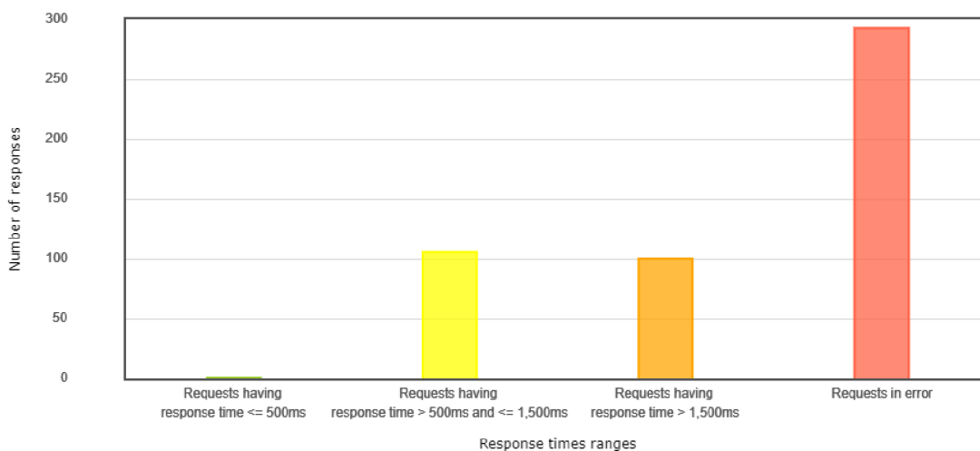
Obr. 3.10: Přehled odezvy ústředny při zatěžování požadavky INVITE.
