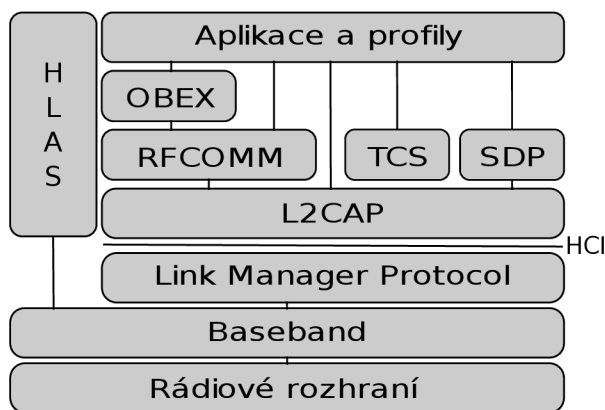
Obrázek 2.1: Bluetooth rozhraní
