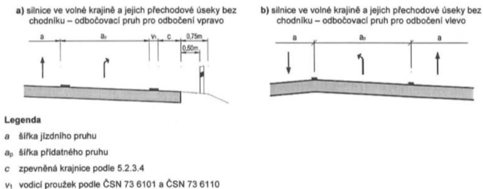
Obrázek 22 – Prvky lemující přídatné pruhy
