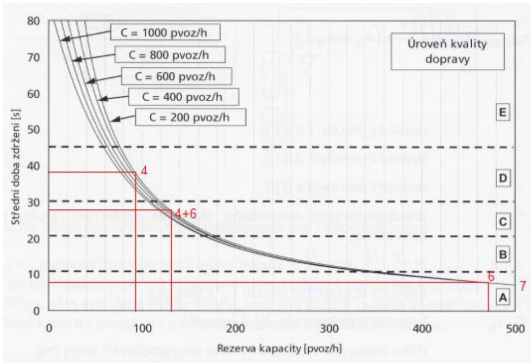
Obrázek 47 vztah střední doby zdržení na kapacitě a její rezervě [TP188]
